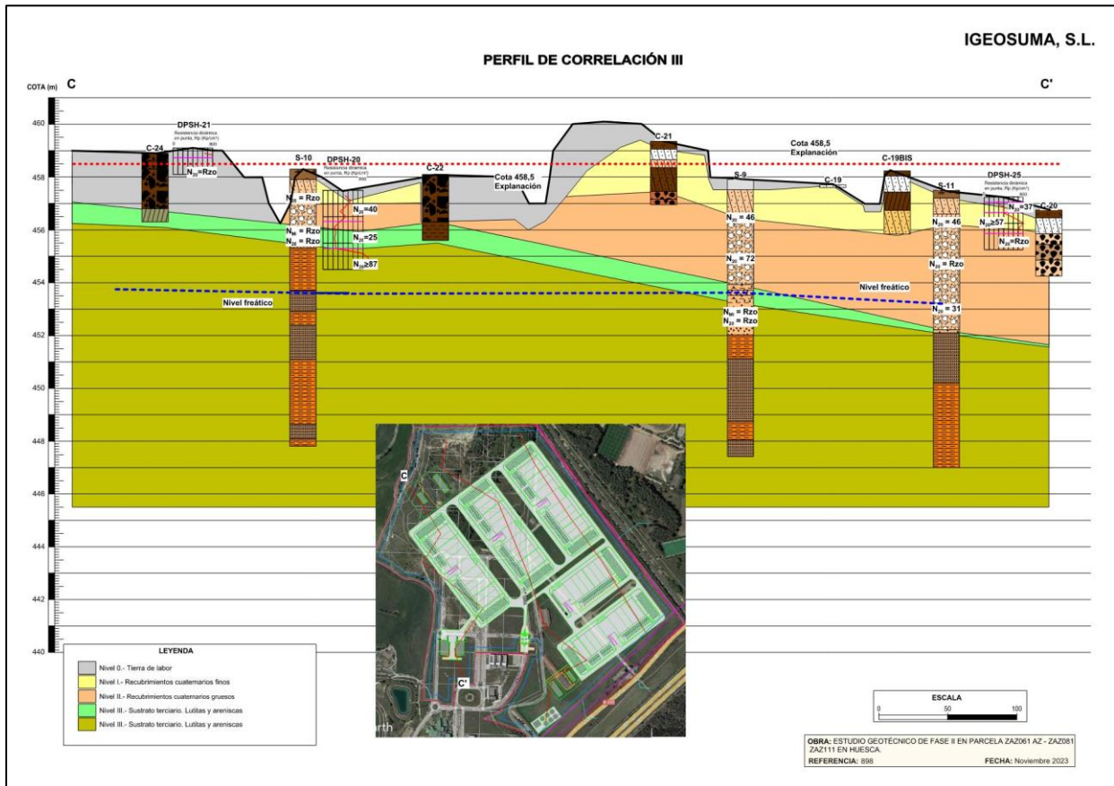
Sección del terreno donde se muestra la geología de la parcela. Fuente: Estudio Geotécnico (Fase 2) en parcela del Parque Tecnológico “Walqa” en T. M. de Huesca. Igeosuma (Noviembre, 2023)
