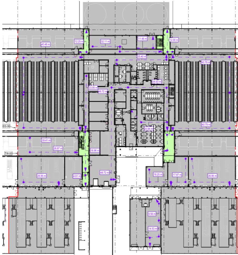
Figura 8. Rutas de evacuación durante la construcción por fases del edificio (Fase 2)
