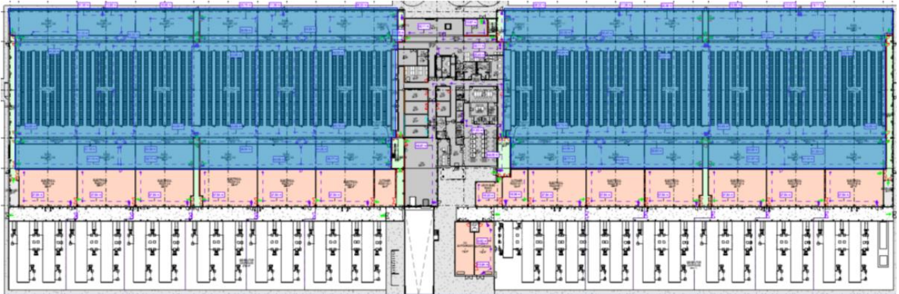
Figura 2. Diagrama de compartimentación de incendios.
