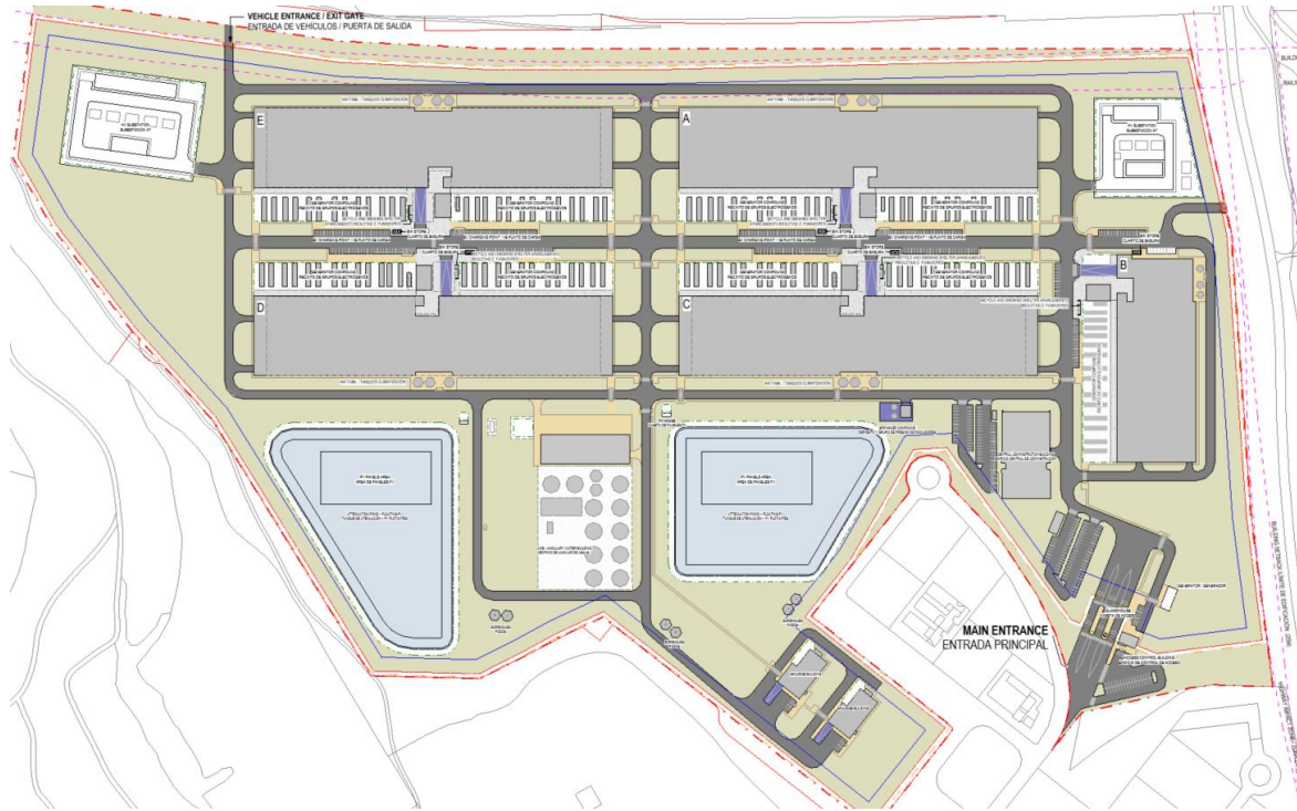
Figura 14. Vías de acceso para servicios de emergencia propuestas en torno a ZAZ081
