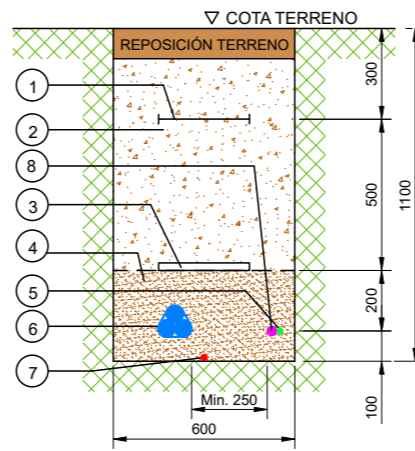
SECCION ZANJA TIPO EN TIERRA 1 LINEA DE M.T. + 1 LINEA DE B.T.
