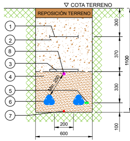
SECCION ZANJA TIPO EN TIERRA 2 LINEAS DE M.T. + 1 LINEA DE B.T.
