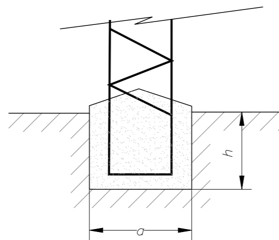
CIMENTACIÓN MONOBLOQUE
