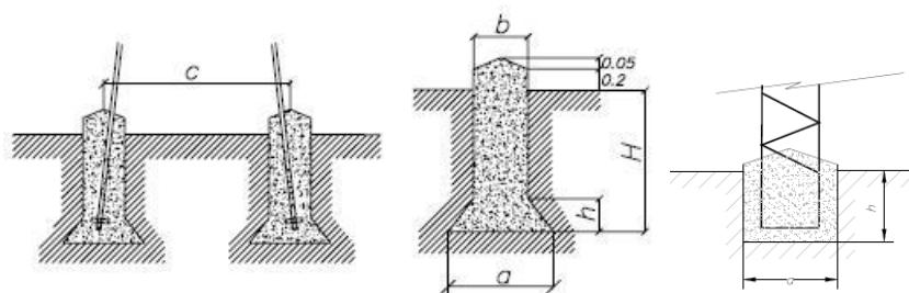
Cimentación tetrablock y monoblock.
