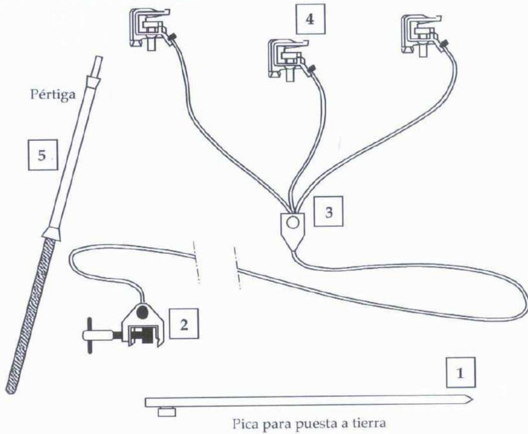
ELEMENTOS DE UN EQUIPO PORTÁTIL DE PUESTA A TIERRA
