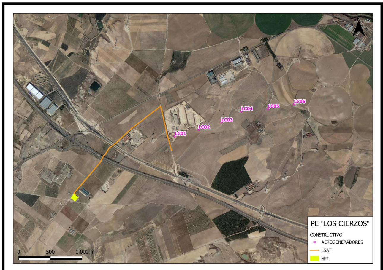
Imagen 1. Constructivo general del Parque Eólico "Los Cierzos".
