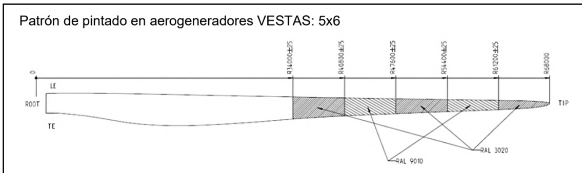
Figura 8: Esquema del patrón de pintado aplicado sobre la pala de los aerogeneradores en PE “El Tollo”
