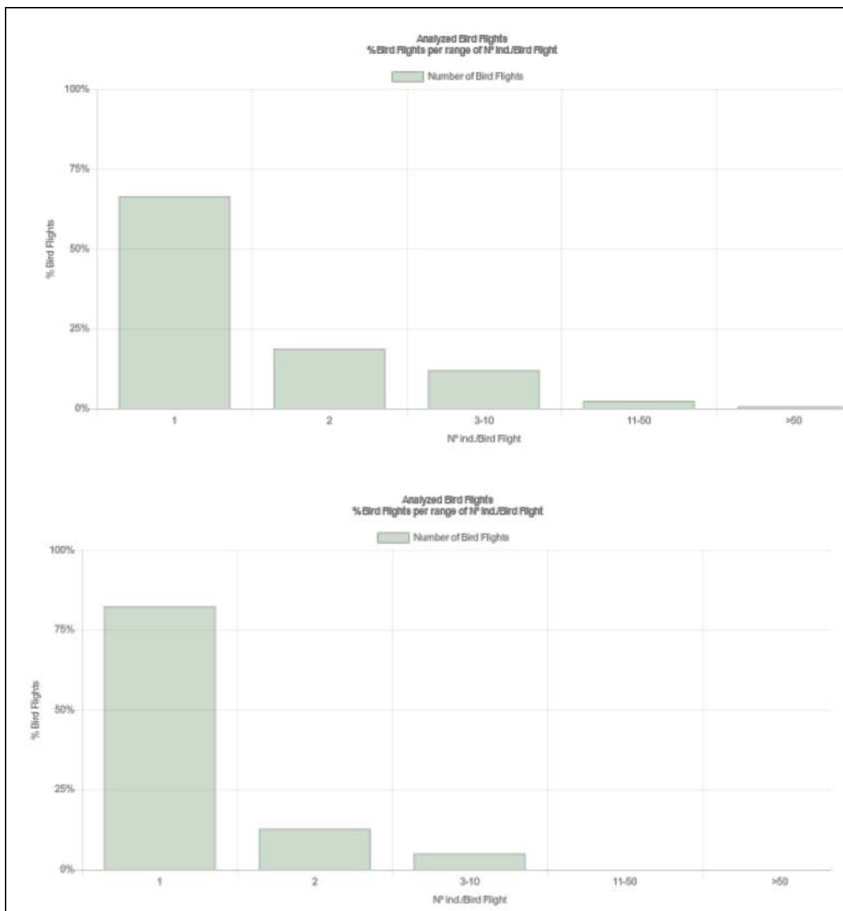
Figura 10. Análisis de vuelo: número de contactos por número de individuos en cada contacto. Aerogenerador A01 y A10.
