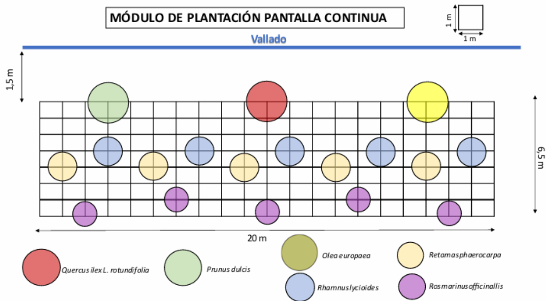
Figura 7 Marco de plantación del apantallamiento vegetal
