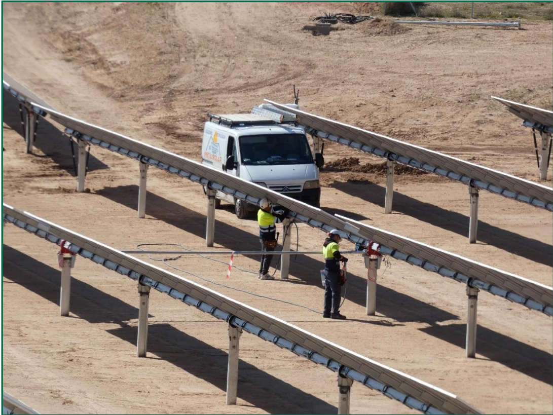
Fotografía 4. Colocación de cableado.
