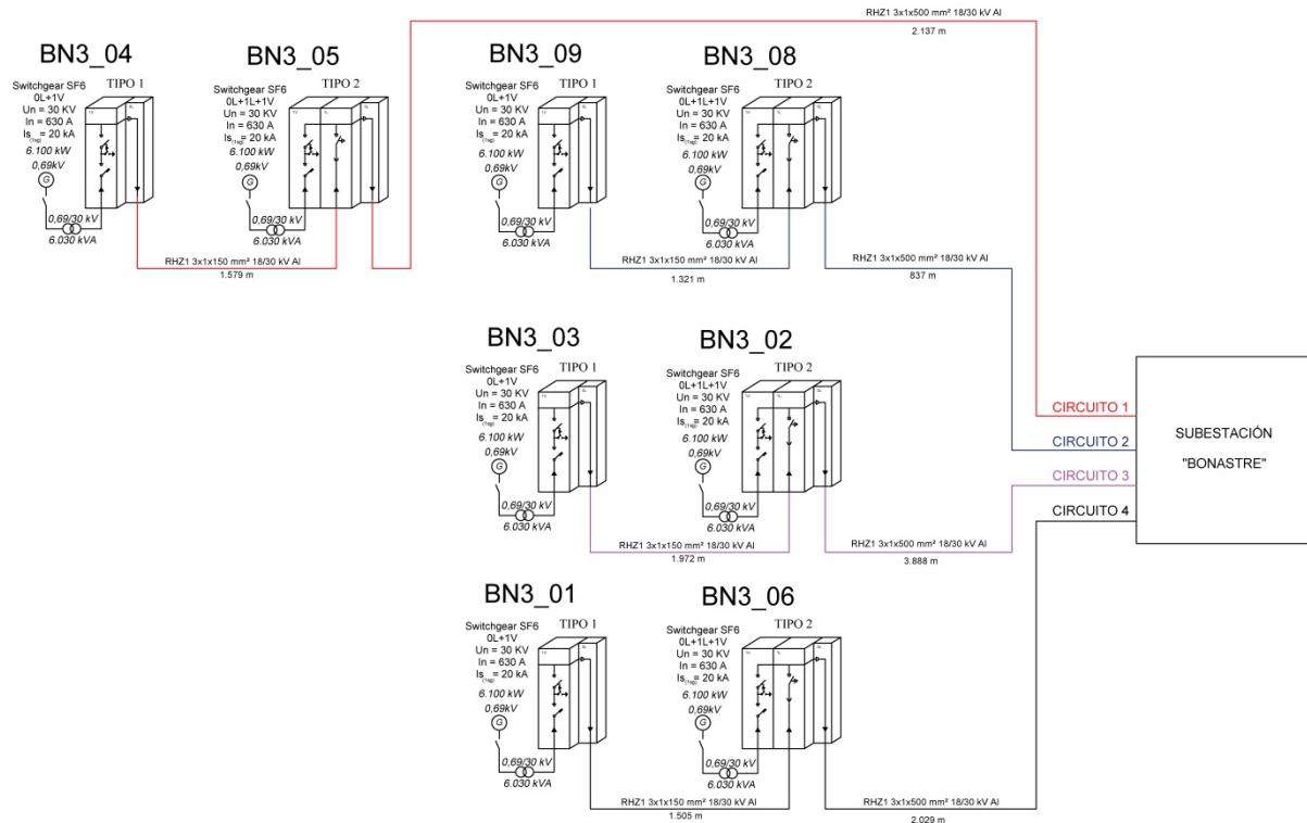
Ilustración 1. Esquema de red eléctrica
