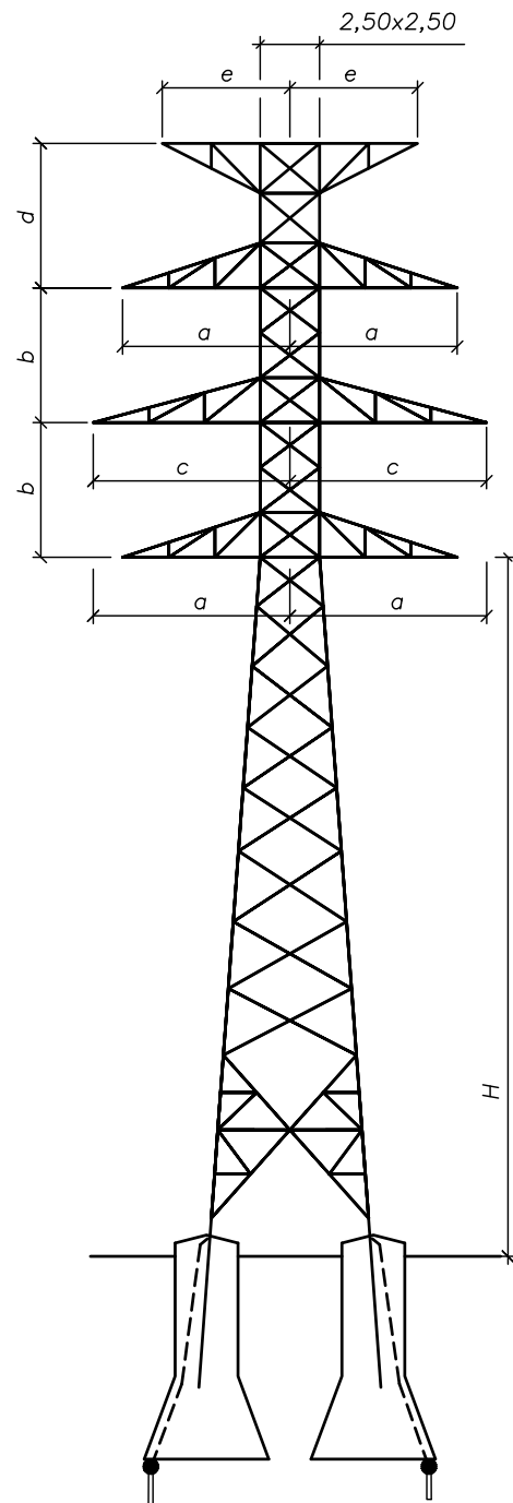
VISTA FRONTAL DESDE APOYO N°2 PARA EL APOYO N°1 VISTA FRONTAL DESDE APOYO N°89 PARA EL APOYO N°90
