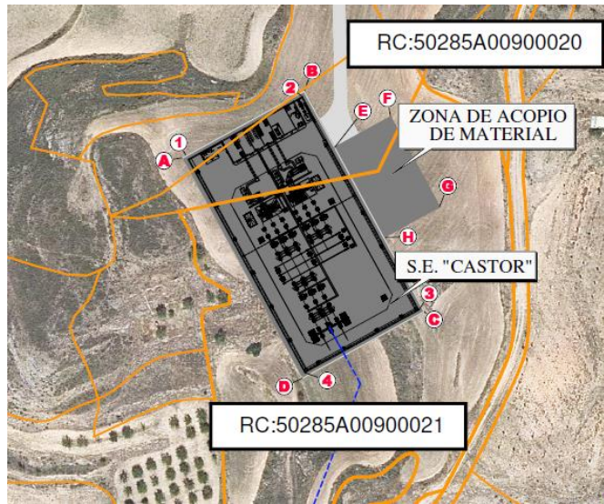
Ilustración 8 Infraestructura de Evacuación - SET Castor
