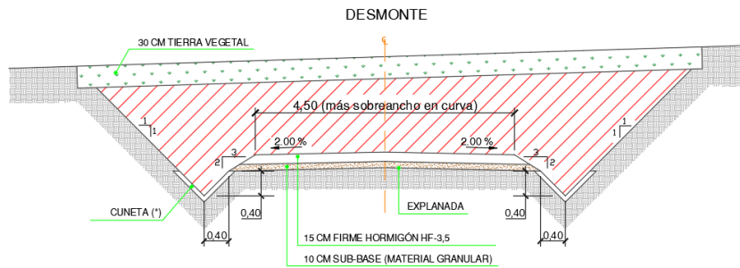
Ilustración 12 Sección tipo viales para pendientes >14%.
