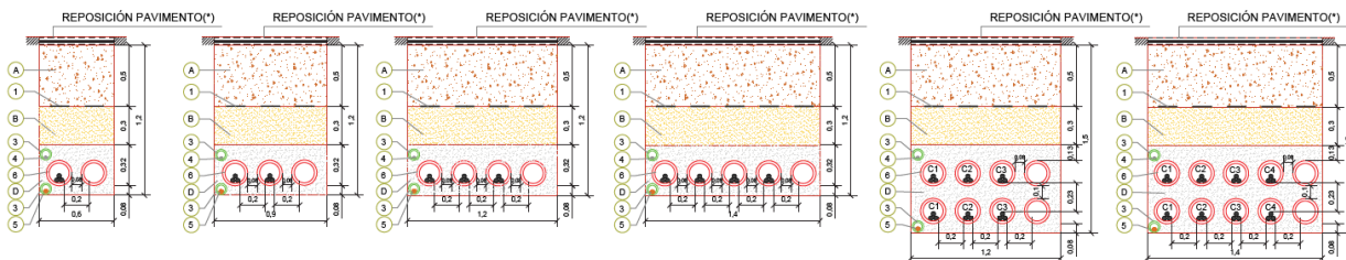
Ilustración 21 Zanjas para circuitos directamente enterrados bajo viales o drenajes.
