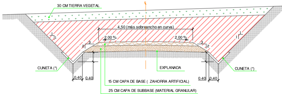
Ilustración 11 Sección tipo viales para pendientes < 10%. Vial primario.
