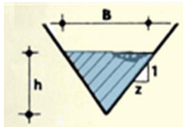
Ilustración 15 Cuneta tipo
