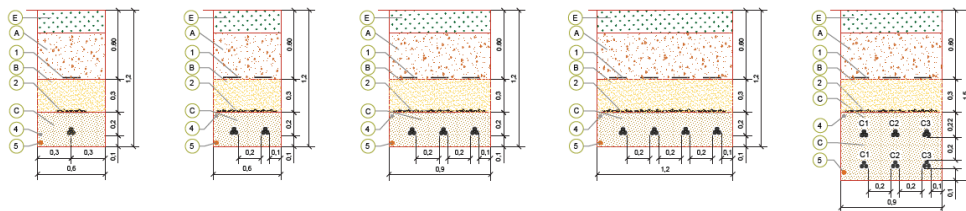
Ilustración 20 Zanjas para circuitos directamente enterrados en terreno agrícola.
