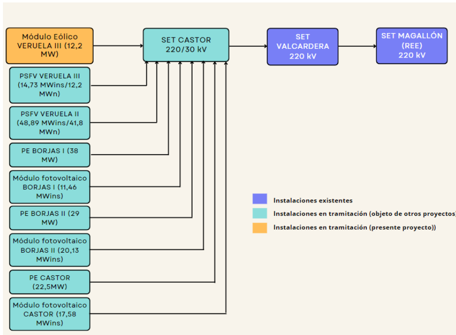
Ilustración 9 Conexión SET Castor
