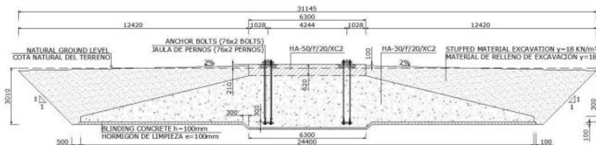
Ilustración 18 Sección de la cimentación: dimensiones establecidas.
