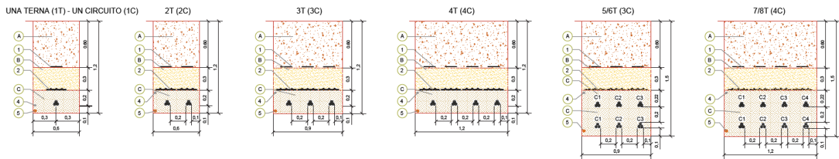
Ilustración 19 Zanjas para circuitos directamente enterrados.
