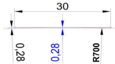
Ilustración 13 Tolerancia irregularidades del suelo.
