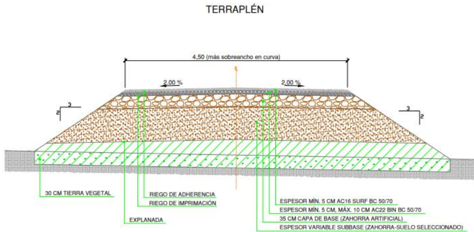
Ilustración 10 Sección tipo vial para pendientes < 10%. Vial Aglomerado
