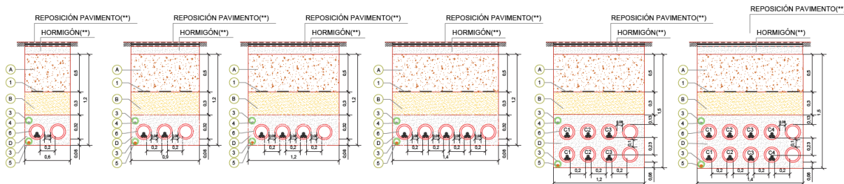
Ilustración 22 Zanjas para circuitos directamente enterrados bajo calzada.
