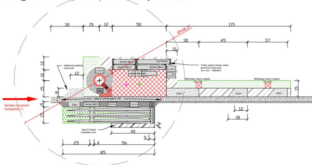
Ilustración 16 Plataforma utilizada / HIBVE3-01
