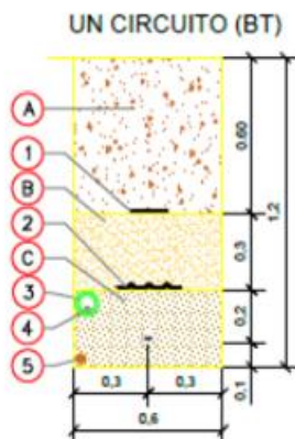
Ilustración 6 Especificación de la zanja de la torre de medición.
