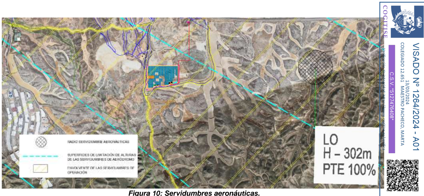
Figura 10: Servidumbres aeronáuticas.
