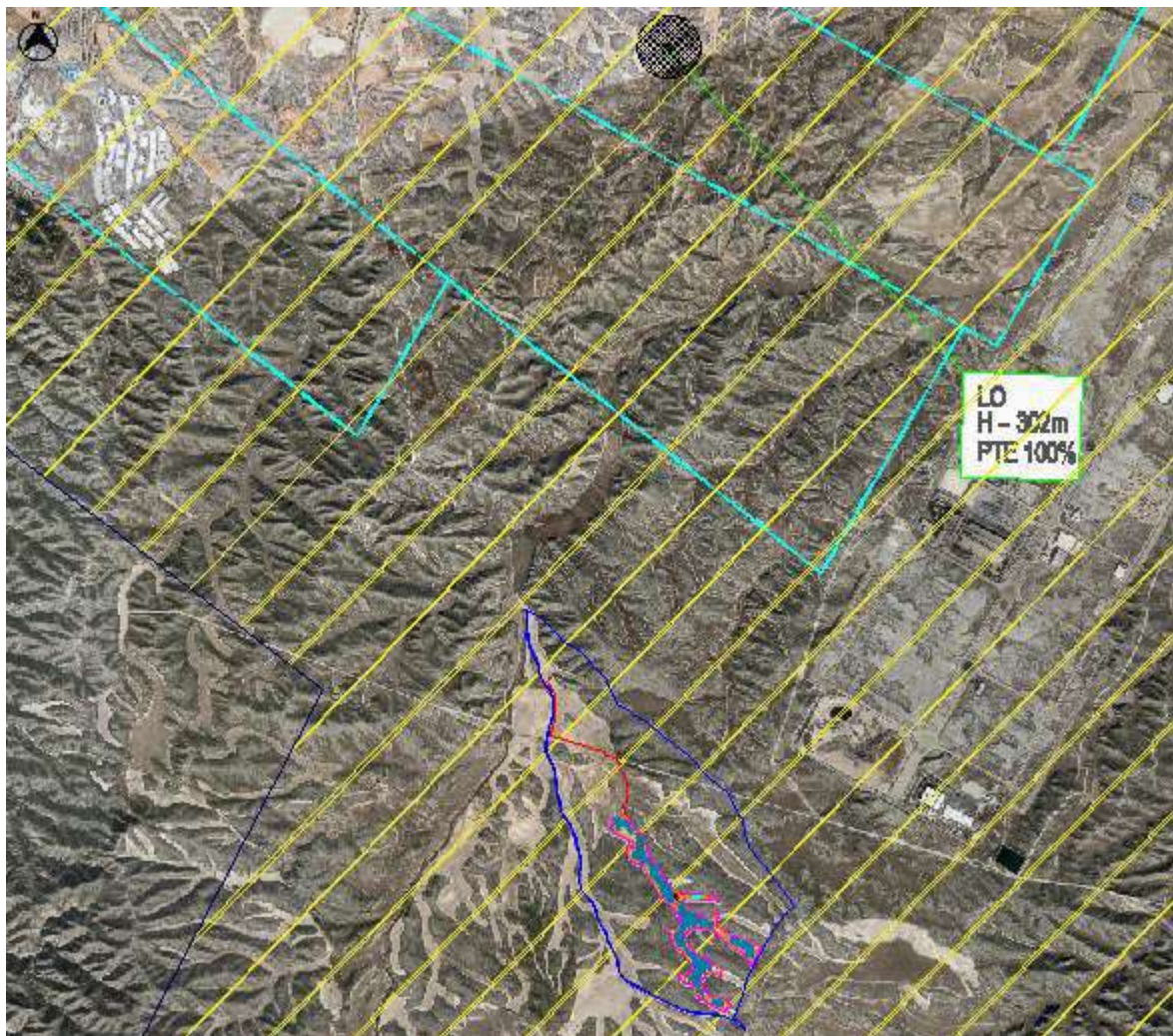
Figura 10: Servidumbres aeronáuticas.
