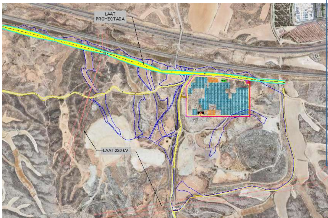
Figura 10: Líneas eléctricas.
