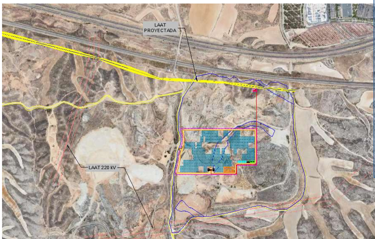
Figura 10: Líneas eléctricas.
