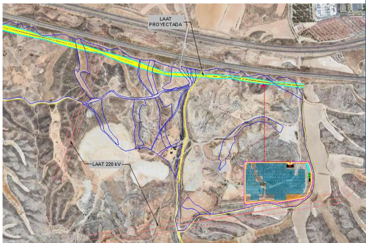
Figura 10: Líneas eléctricas.
