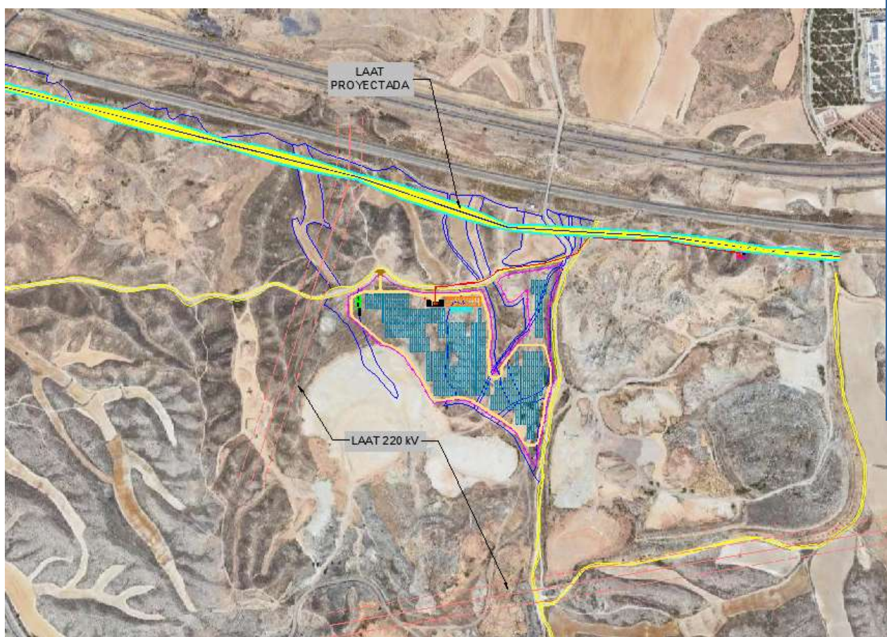
Figura 10: Líneas eléctricas.
