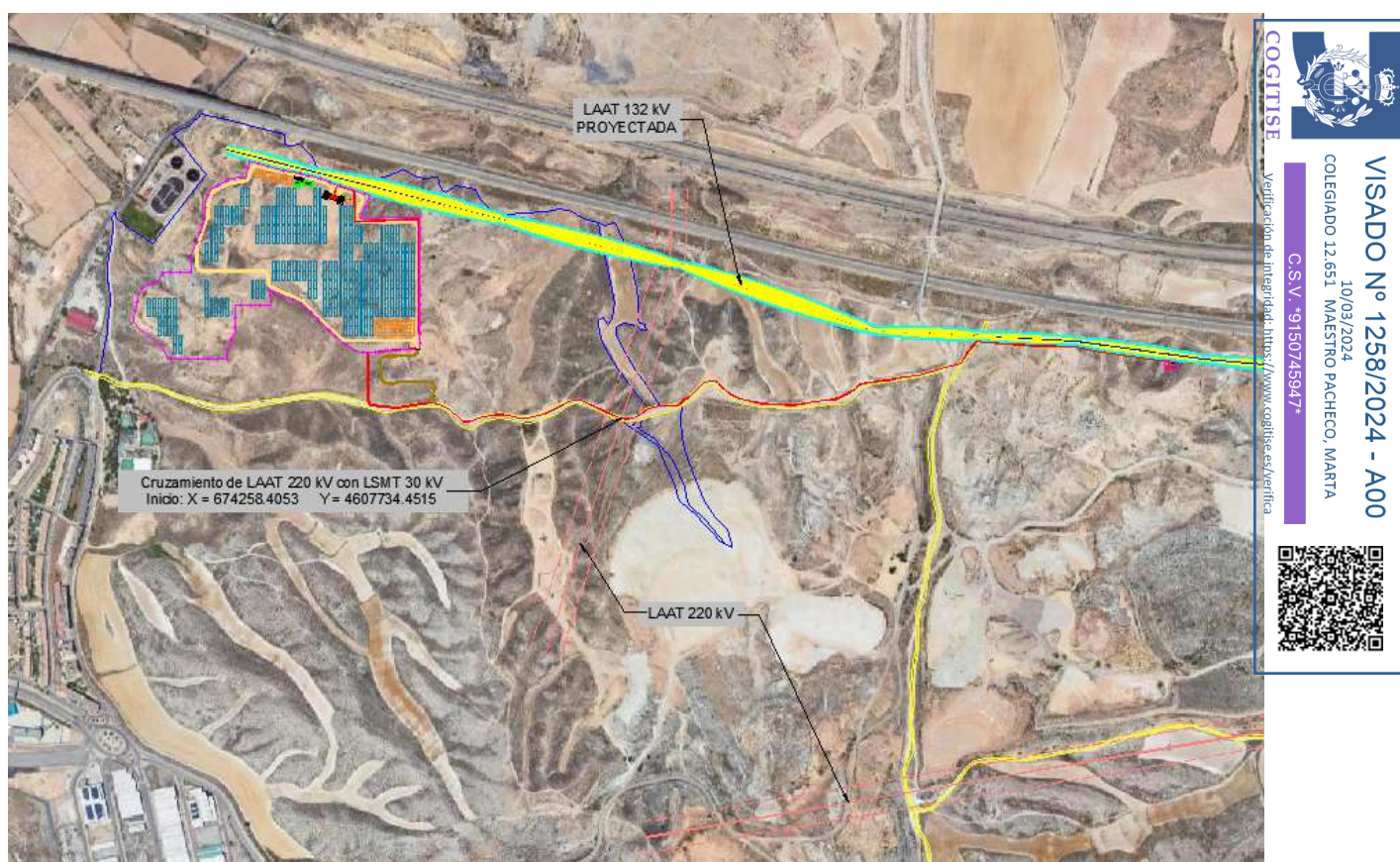
Figura 10: Líneas eléctricas.
