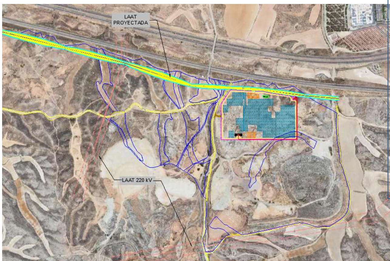
Figura 10: Líneas eléctricas.
