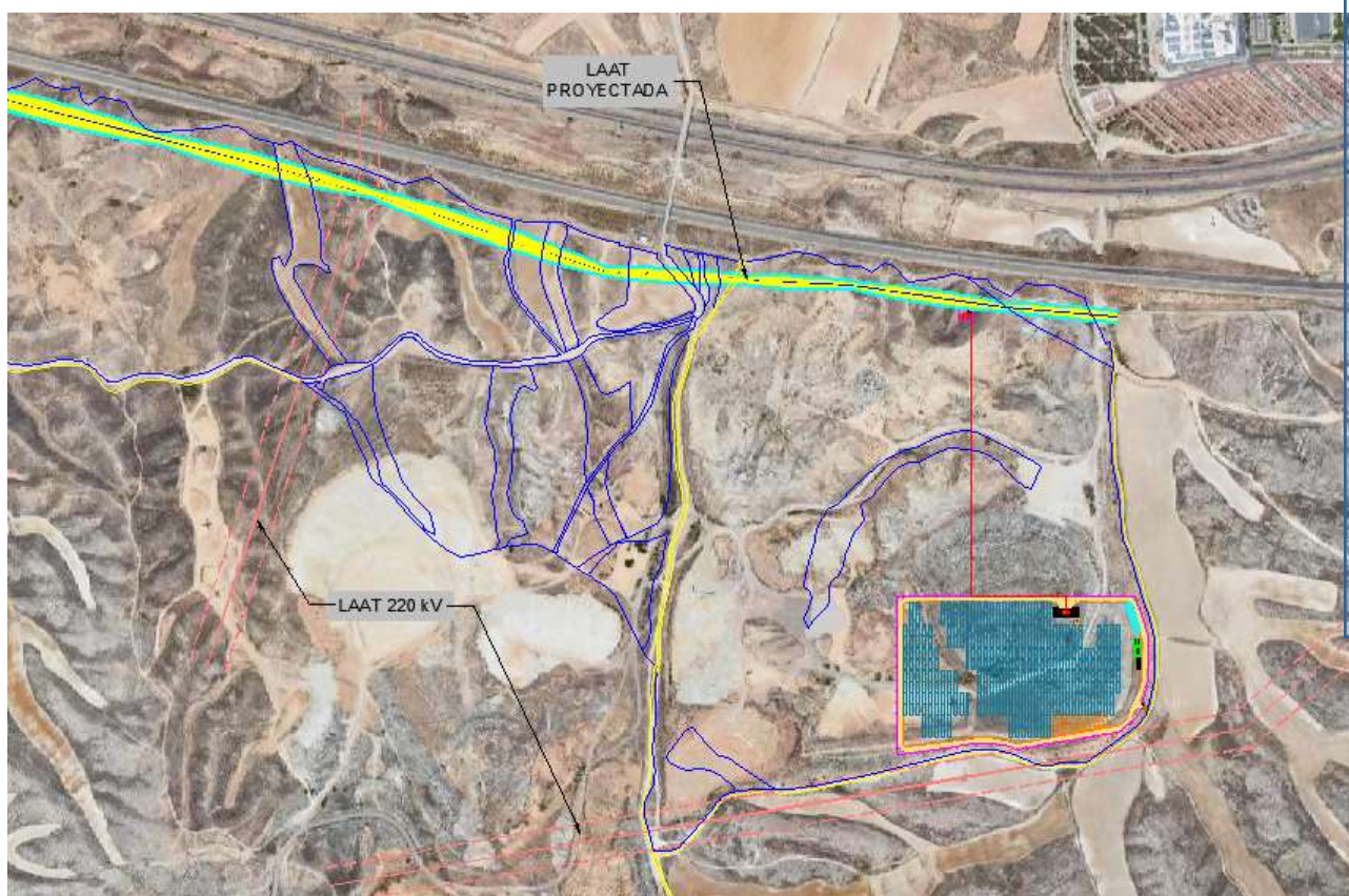
Figura 10: Líneas eléctricas.
