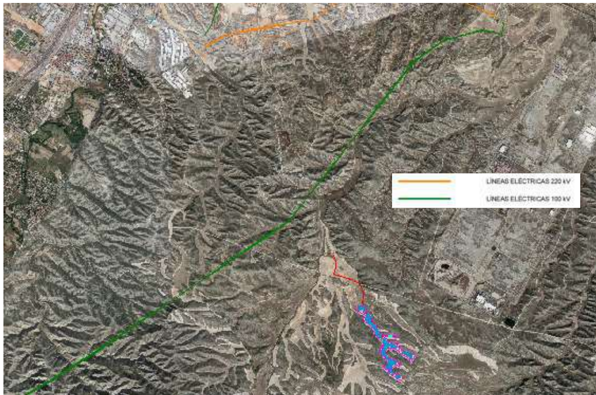
Figura 10: Mapa de líneas eléctricas.
