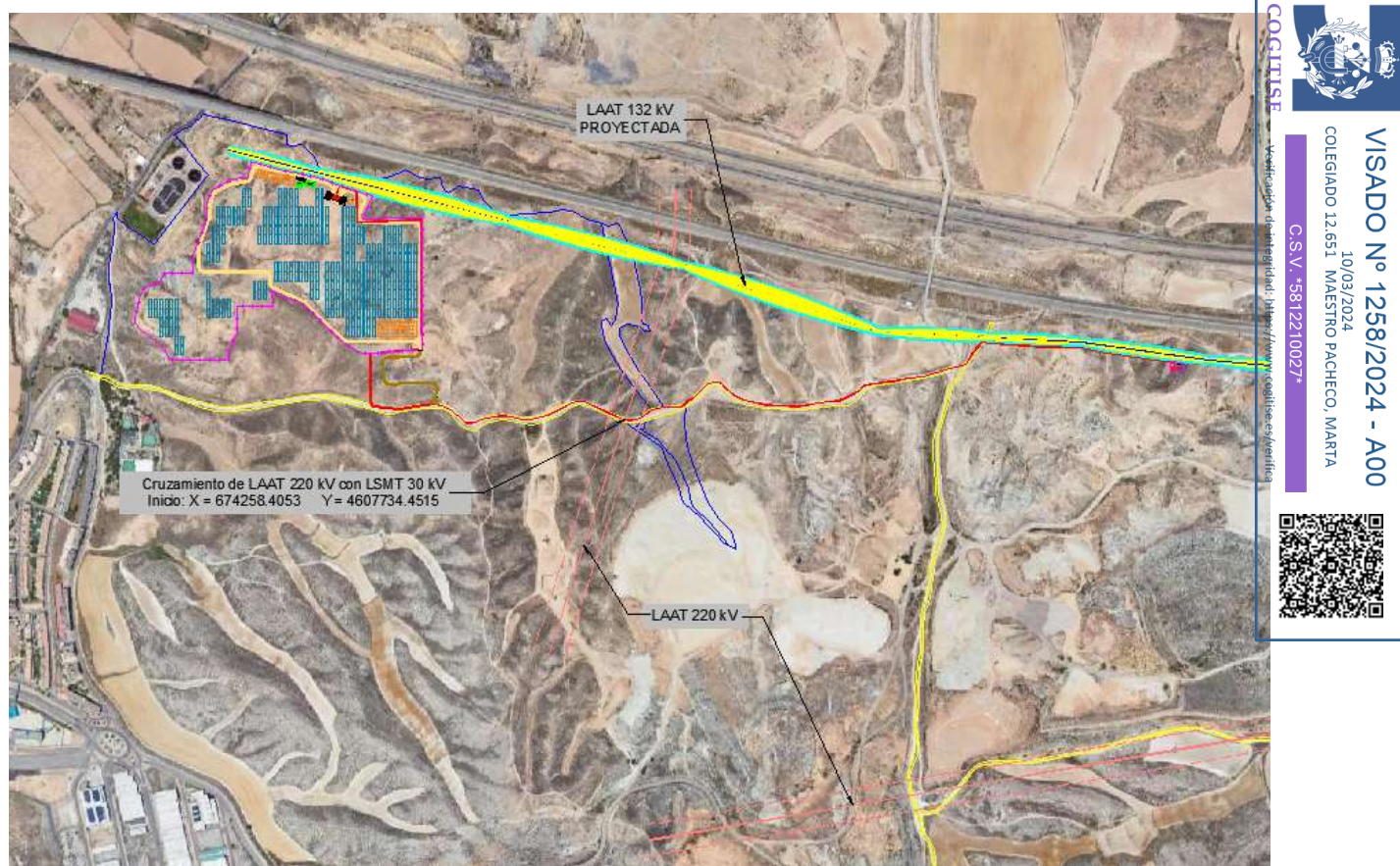
Figura 10: Líneas eléctricas.
