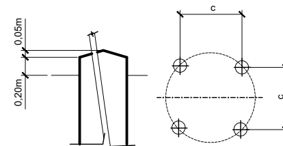
DETALLE A
