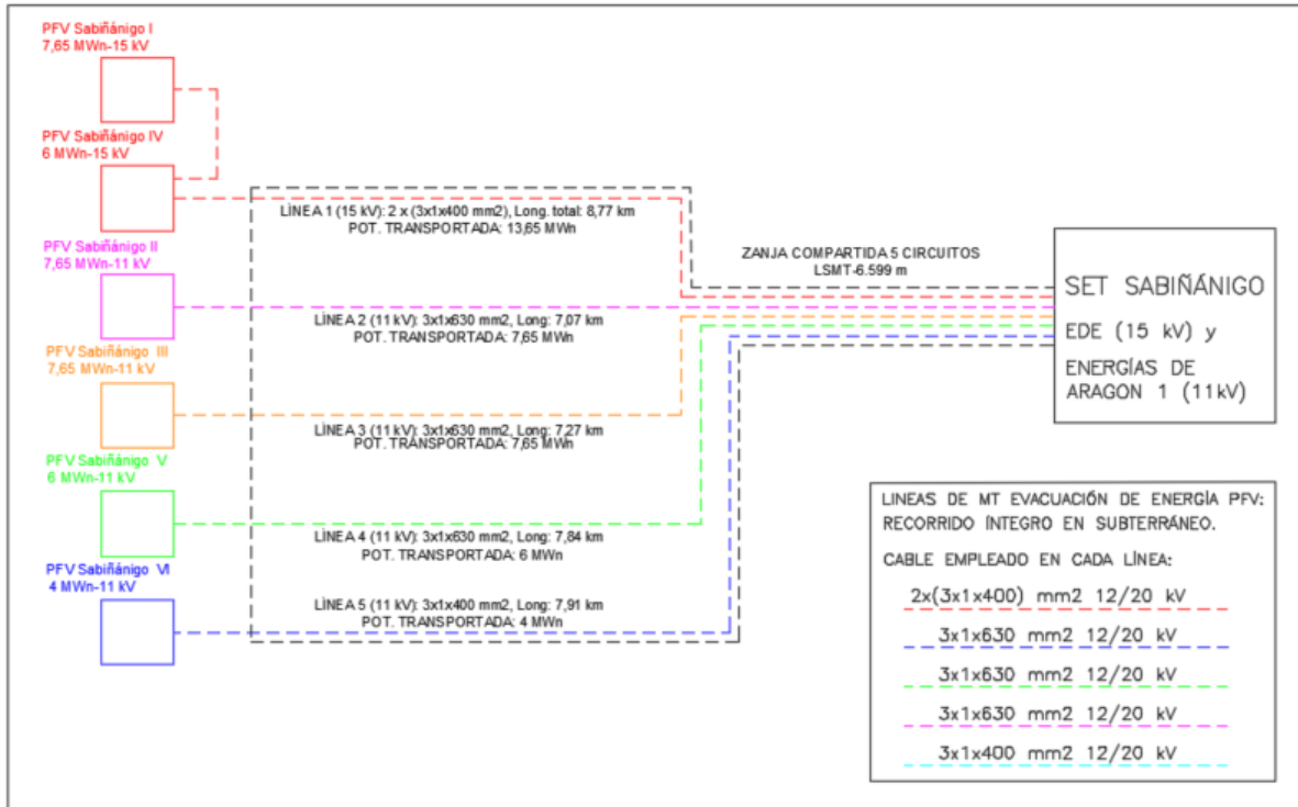
6 PLANTAS FV Y 5 LINEAS SUBTERRANEAS DE MEDIA TENSIÓN
