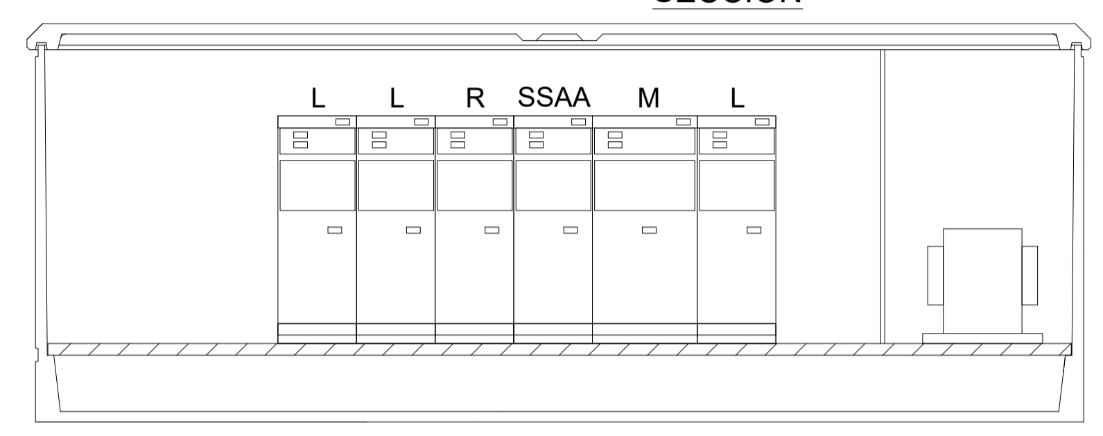
SECCIÓN
