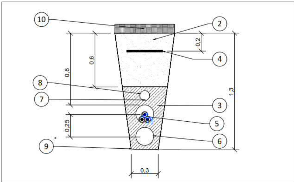
Figura 5: Colocación de cables en tresbolillo.
