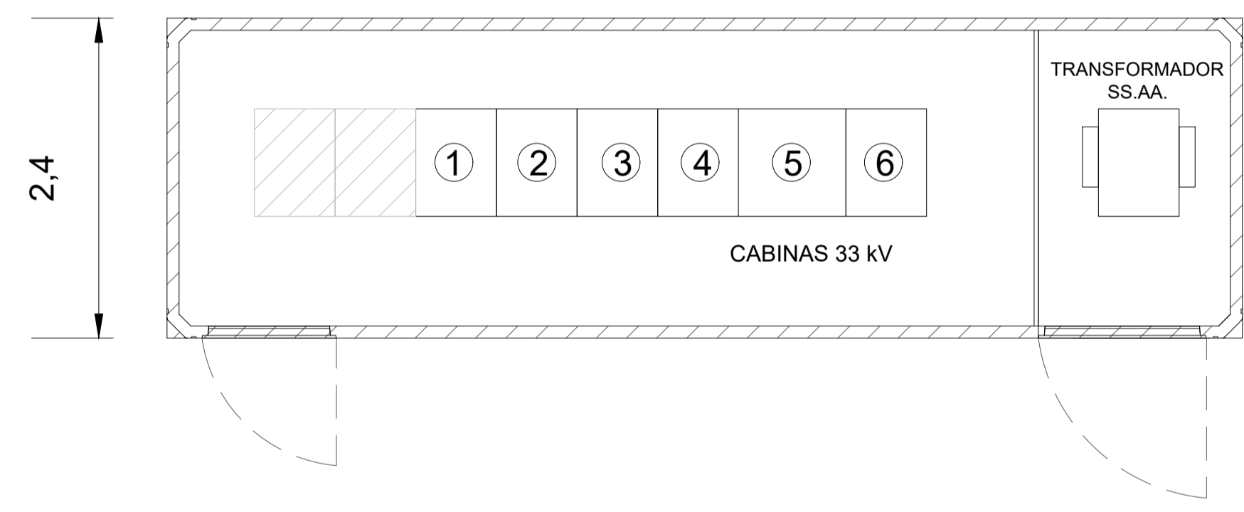
VISTA PLANTA
