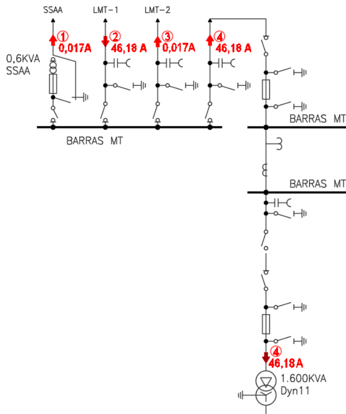
Fig. 2: Unifilar nivel de tensión 20kV con intensidades consideradas
