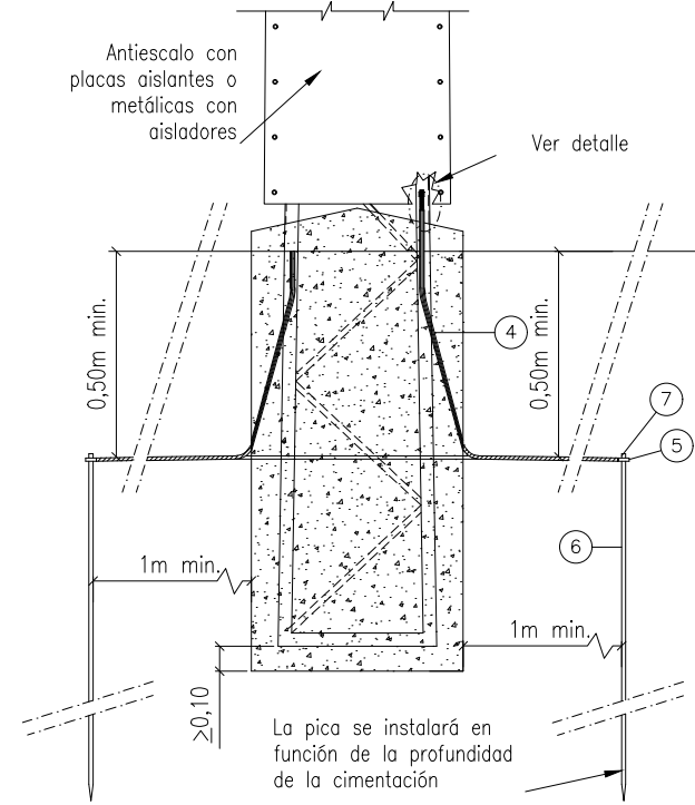
SECCIÓN B-B
