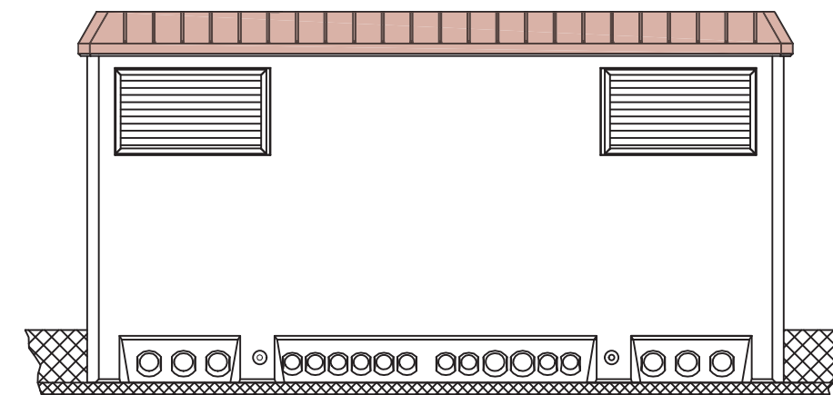
VISTA POSTERIOR
