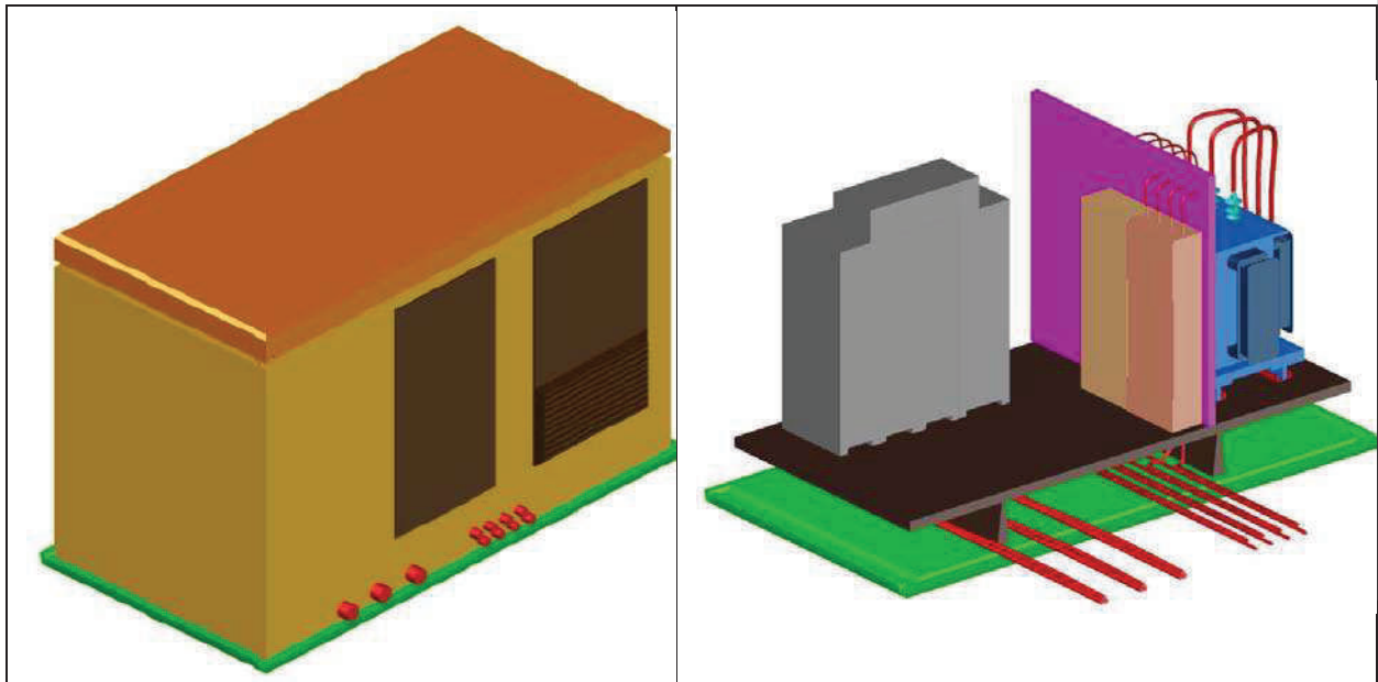
Fig. 1: Vistas 3D Centro transformación tipo en edificio prefabricado de superficie, 24 kV. un trafo.
