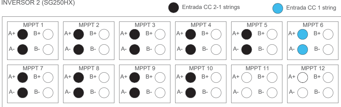
MPPT 1 al 5, y 7 al 10
