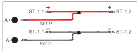
MPPT 1 al 5, y 7 al 10
