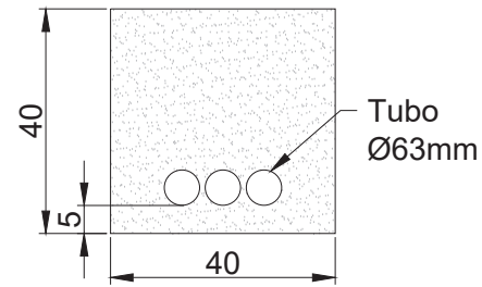
ZANJA STRING-3
