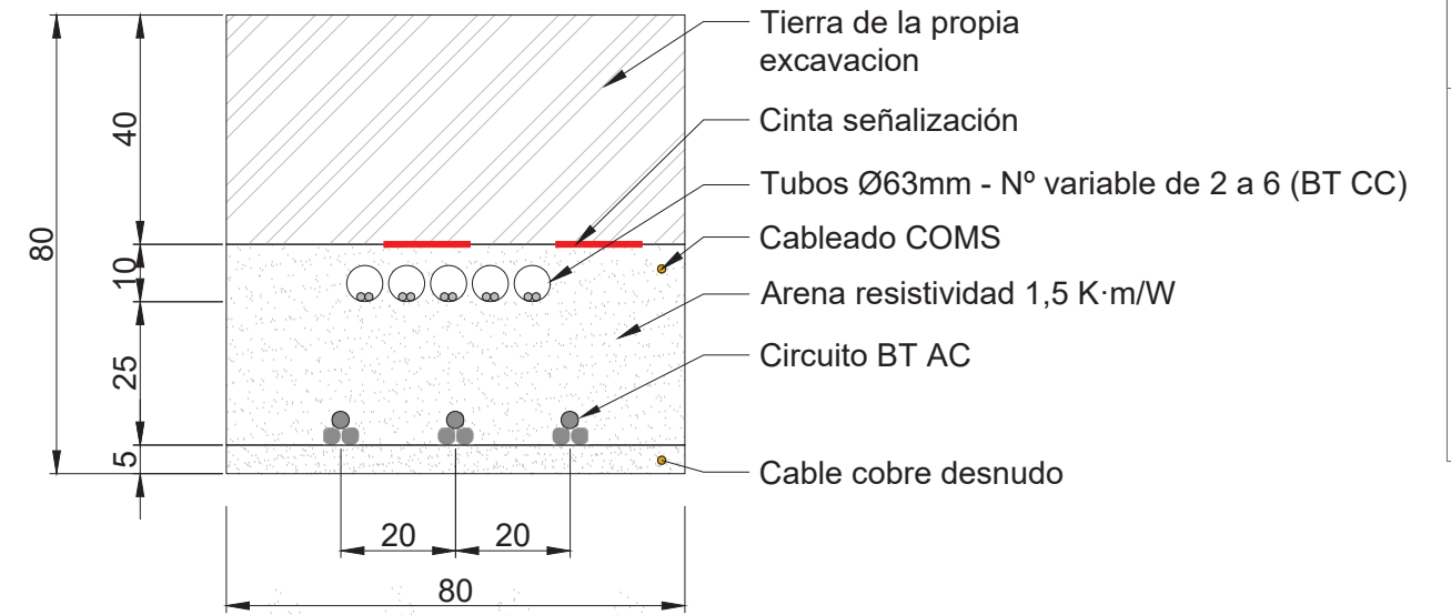
ZANJA COMPARTIDA (SRTRING - N3)
