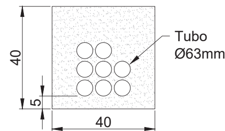
ZANJA STRING-8
