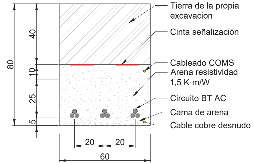
ZANJA N3 - 3
