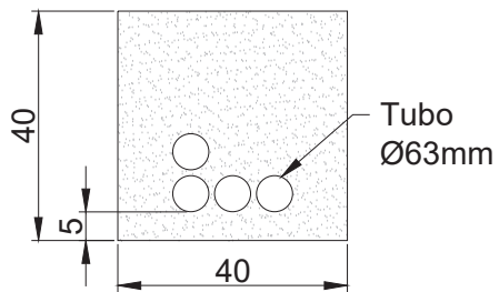
ZANJA STRING-4
