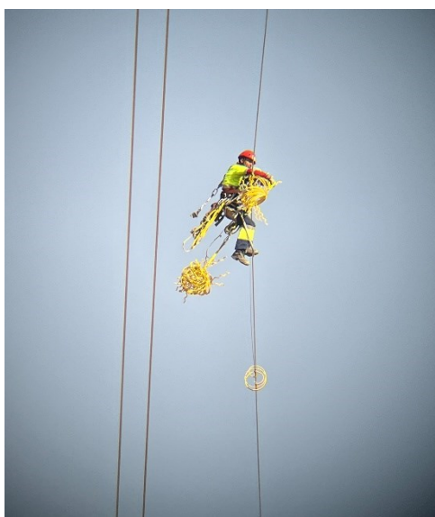
Figura 4 Colocación cable de los protectores para aves
