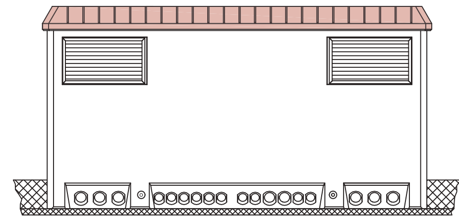
VISTA POSTERIOR
