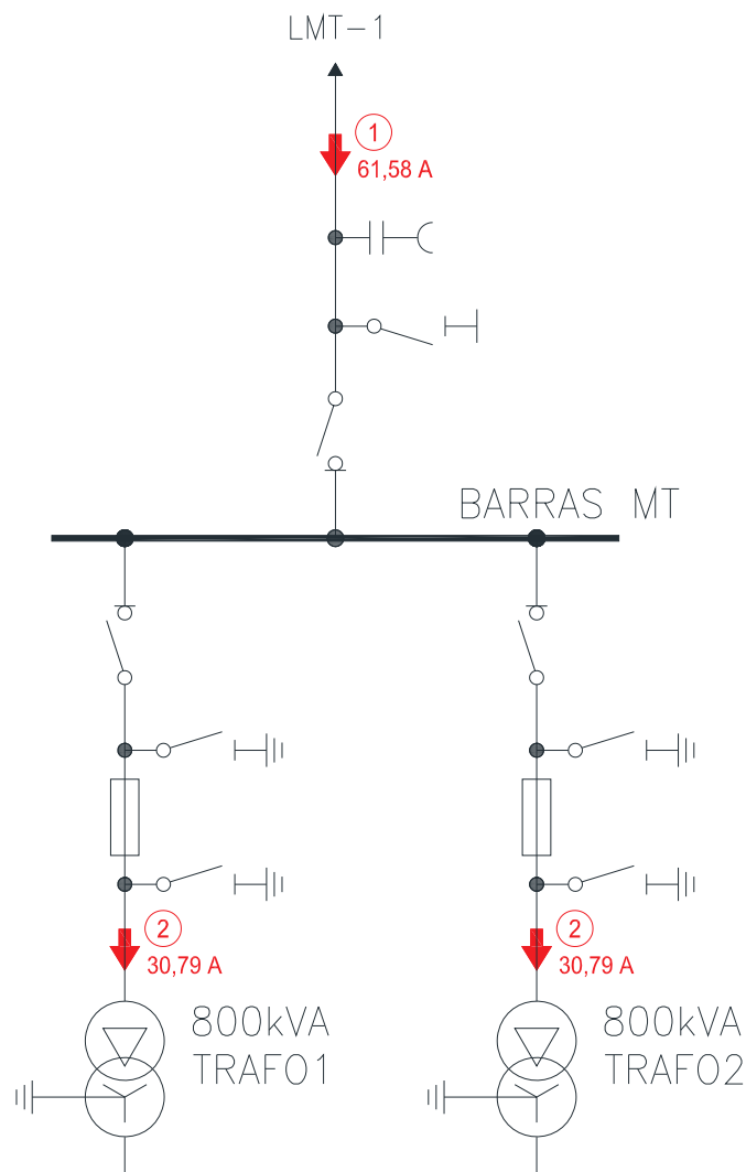
Unifilar nivel de tensión 15kV con intensidades consideradas
