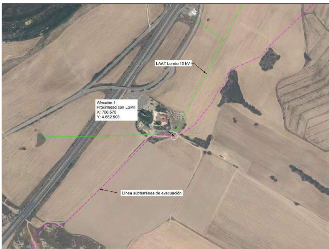
Ilustración 3: afecciones LSMT PFV La Mallata sobre la LAMT Loreto 115 kV (proximidad)
