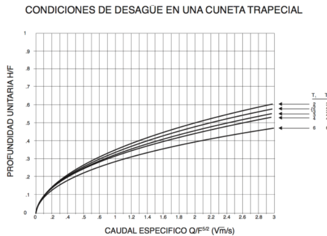
Figura 31.- Diagrama Profundidad-caudal
