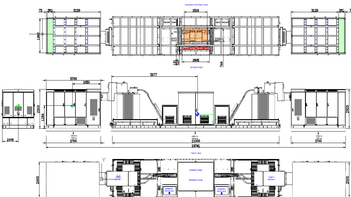
Figura 38.- Vista 1. Ejecución SKID POWER ELECTRONICS FS3510K
