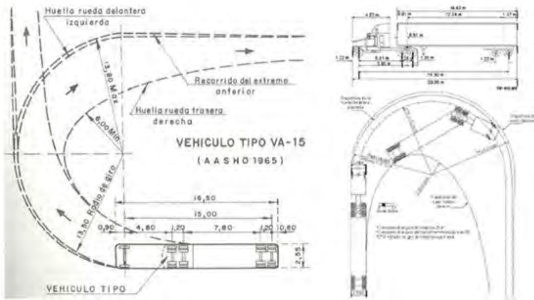
Figura 36.- Esquemas de giro tipo VA-15 según AASTHO
