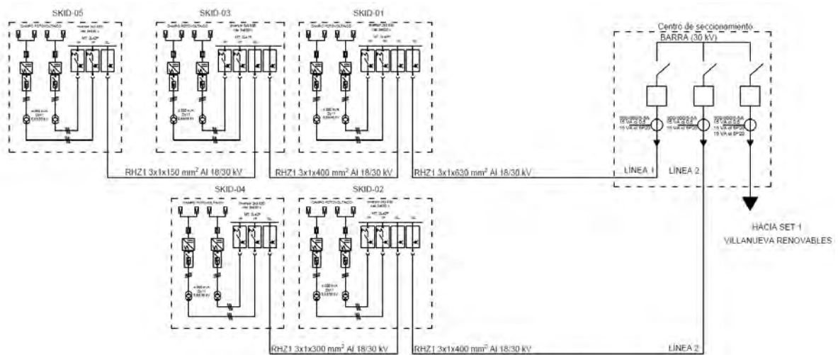
Figura 10.- Esquema interconexión MT
