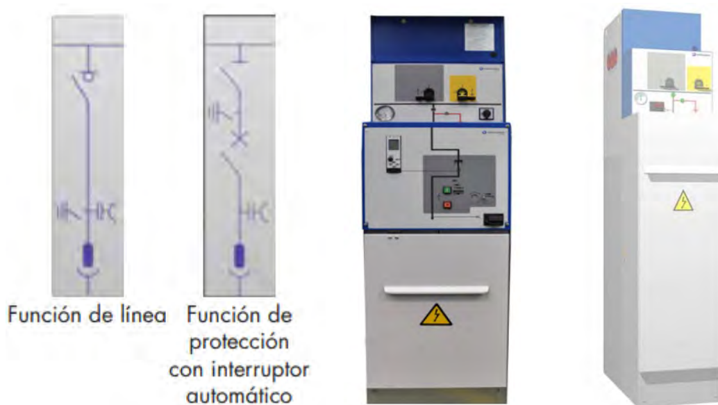
Figura 21.- Esquema unifilar celdas de MT
