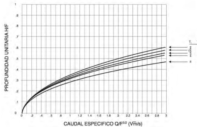
Figura 35.- Diagrama Profundidad-caudal
