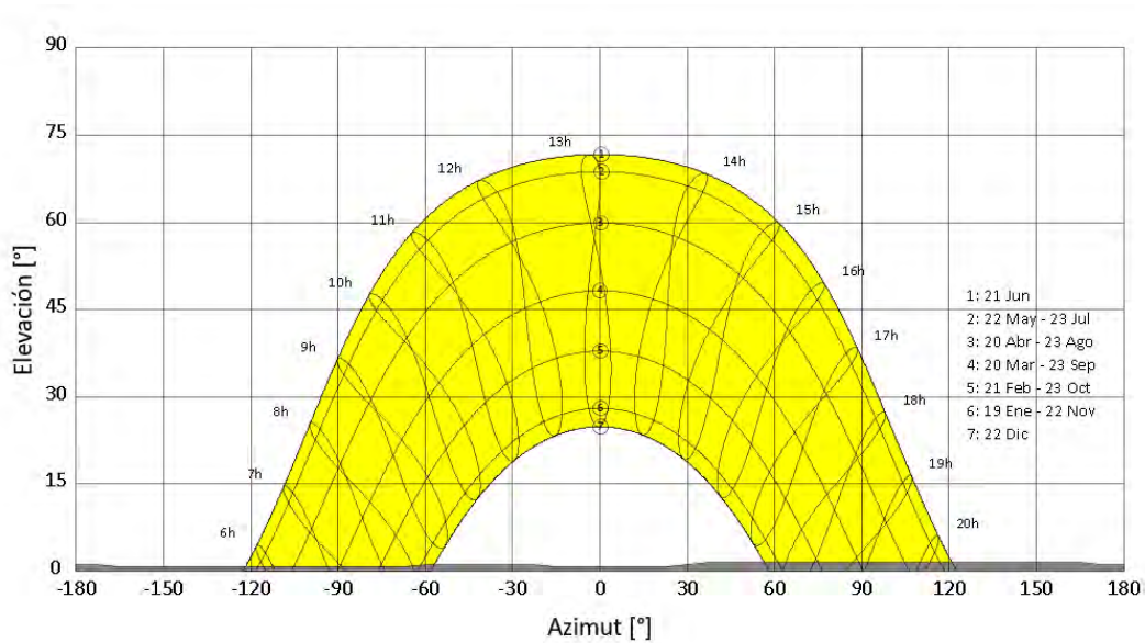
Figura 5: Perfil del horizonte (fuente datos: PVGIS 5)
