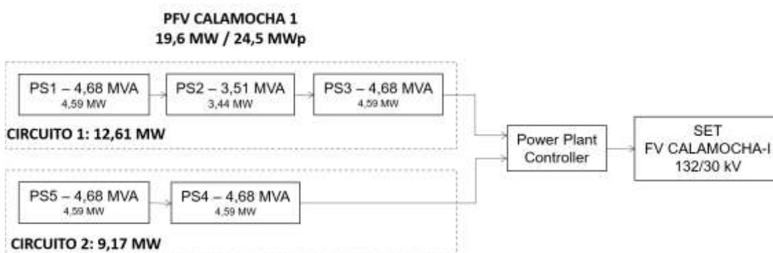
Ilustración 9: Esquema de conexión de la red de MT del PFV
