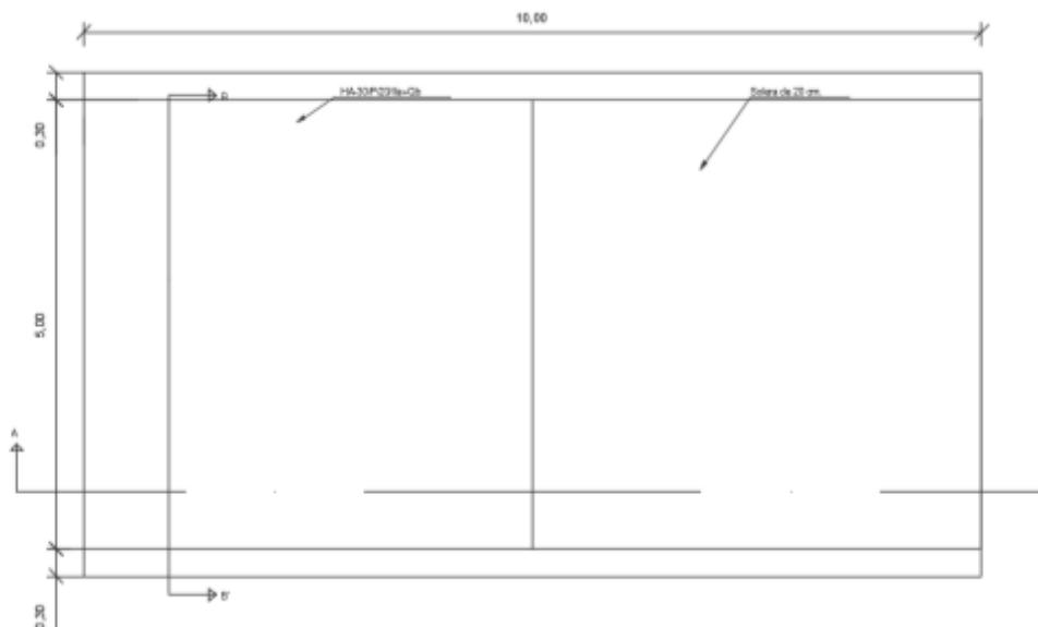
Ilustración 5: Losa de hormigón armado
