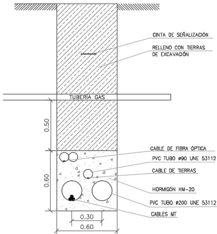
Ilustración 4: Zanja tipo cruzamiento LSMT y Gasoducto
