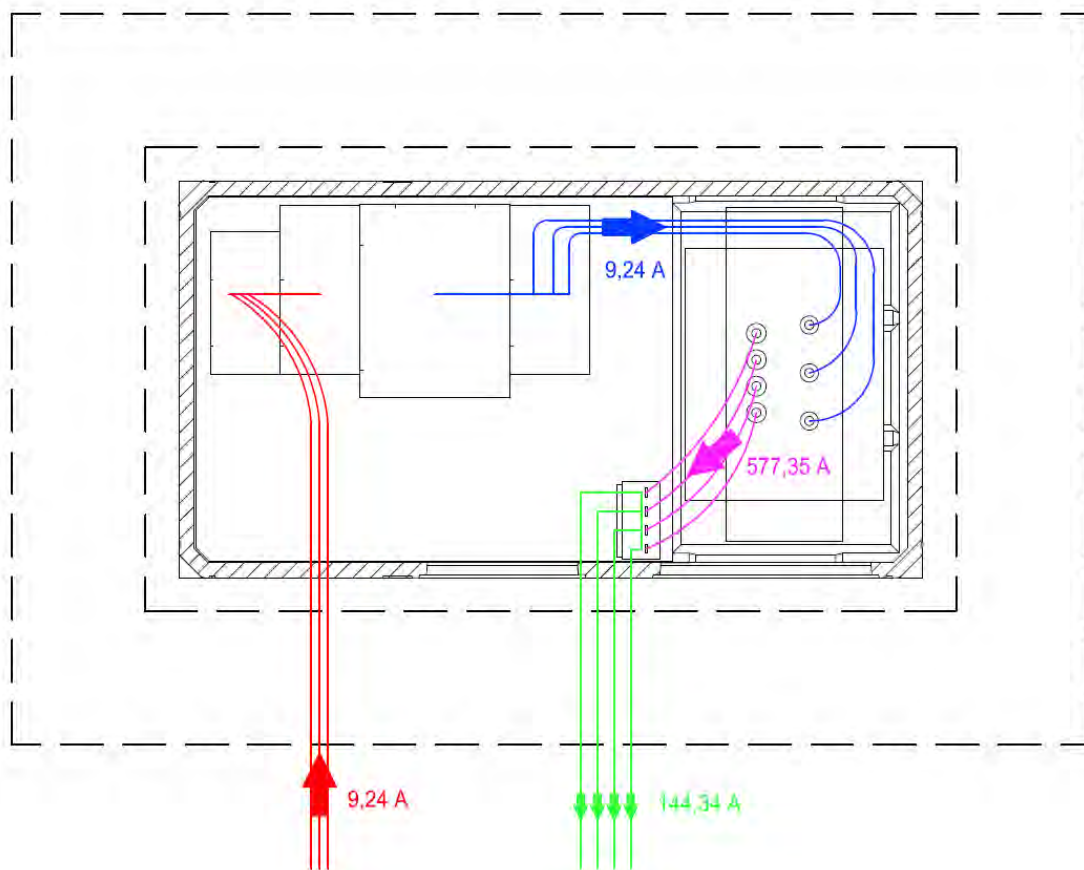
Fig. 4 Intensidades para cálculo de campo magnético.
