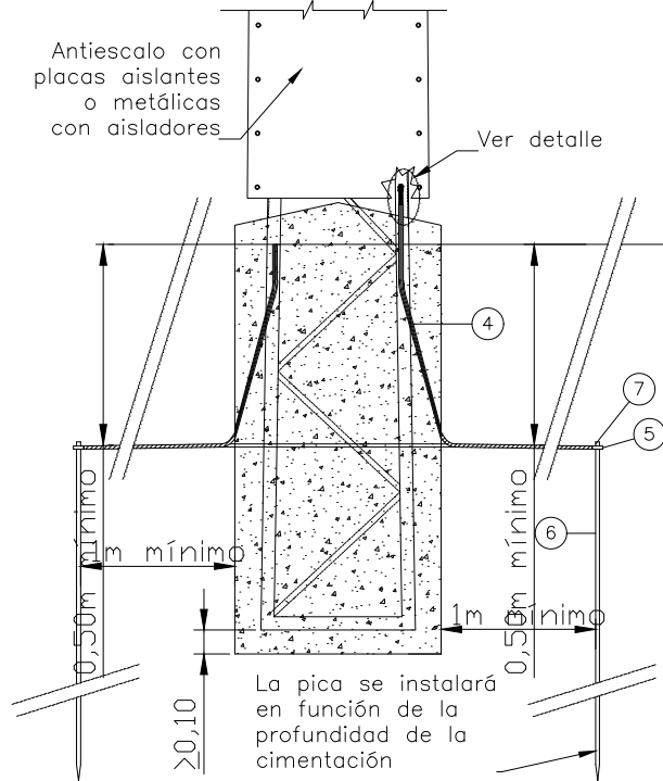
SECCIÓN B-B
