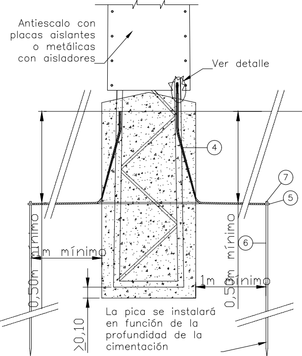
SECCIÓN A-A
