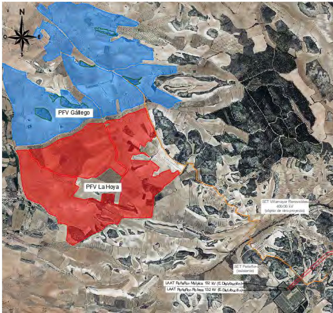
Ilustración 2: Afección RSMT Gállego y La Hoya con LAAT 132 kV Aliagar – Peñaflor
