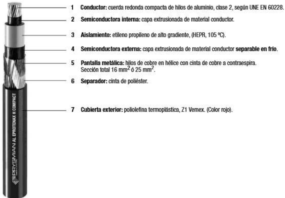
Figura 10. Componentes de conductor de la línea de evacuación
