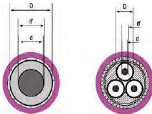
Figura 11. Diámetro de cuerda y semi interior del cable de la línea de evacuación
