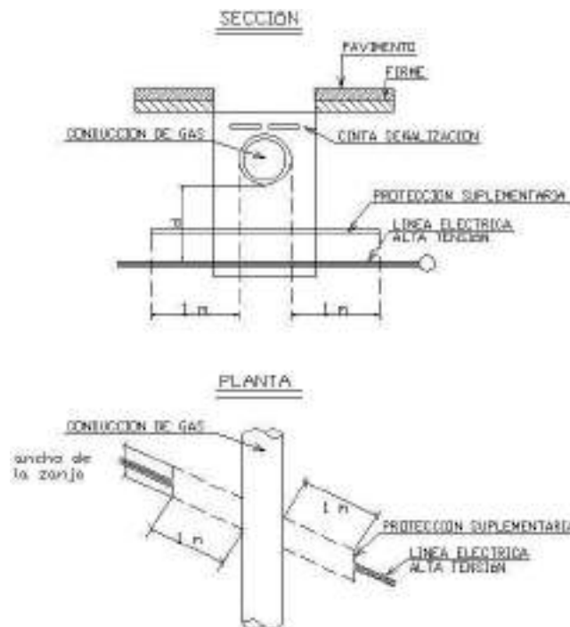
Figura 16. Canalización de gas
