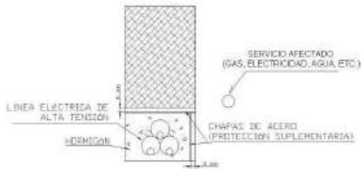
Figura 17. Canalización de cables de energía
