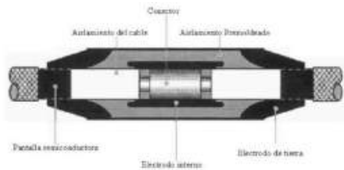
Figura 14. Figura de empalmes premoldeados
