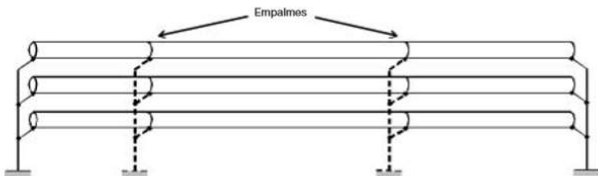
Figura 13. Esquema de conexión rígida a tierra
