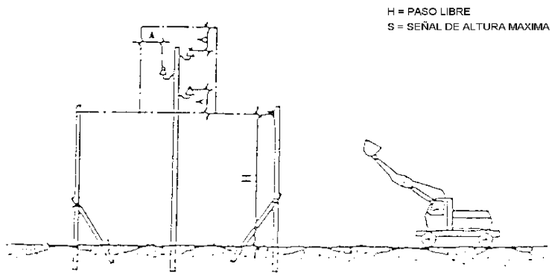
PÓRTICO DE BALIZAMIENTO EN LÍNEAS ELÉCTRICAS AÉREAS
