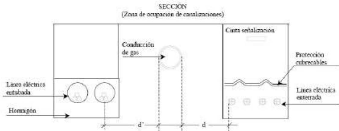
Sección (Zona de ocupación de canalizaciones)
