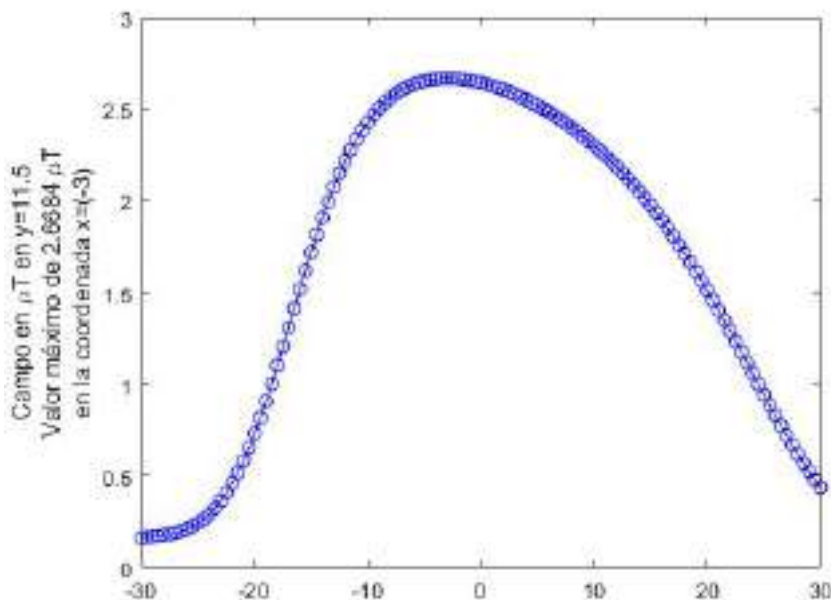
Figura 5: Representación del campo a 1 metro vallado en sentido NORTE.
