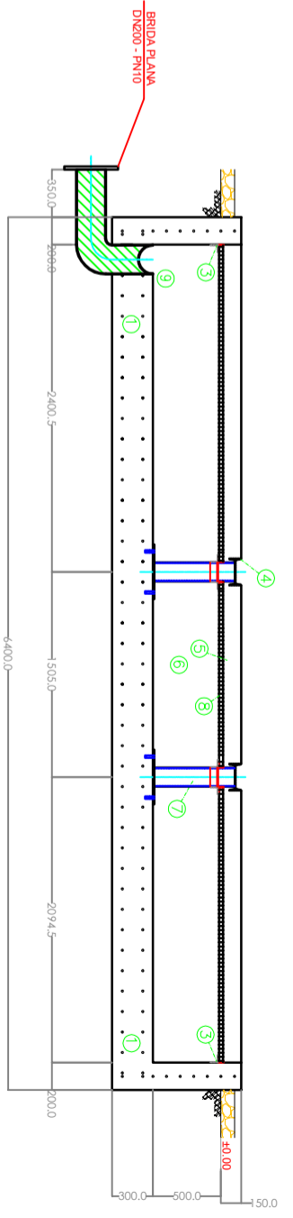
SECCIÓN B-B
