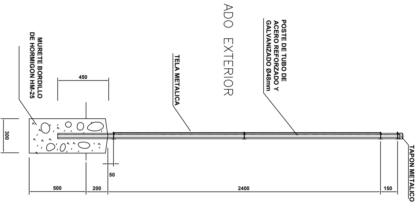
PERFIL
