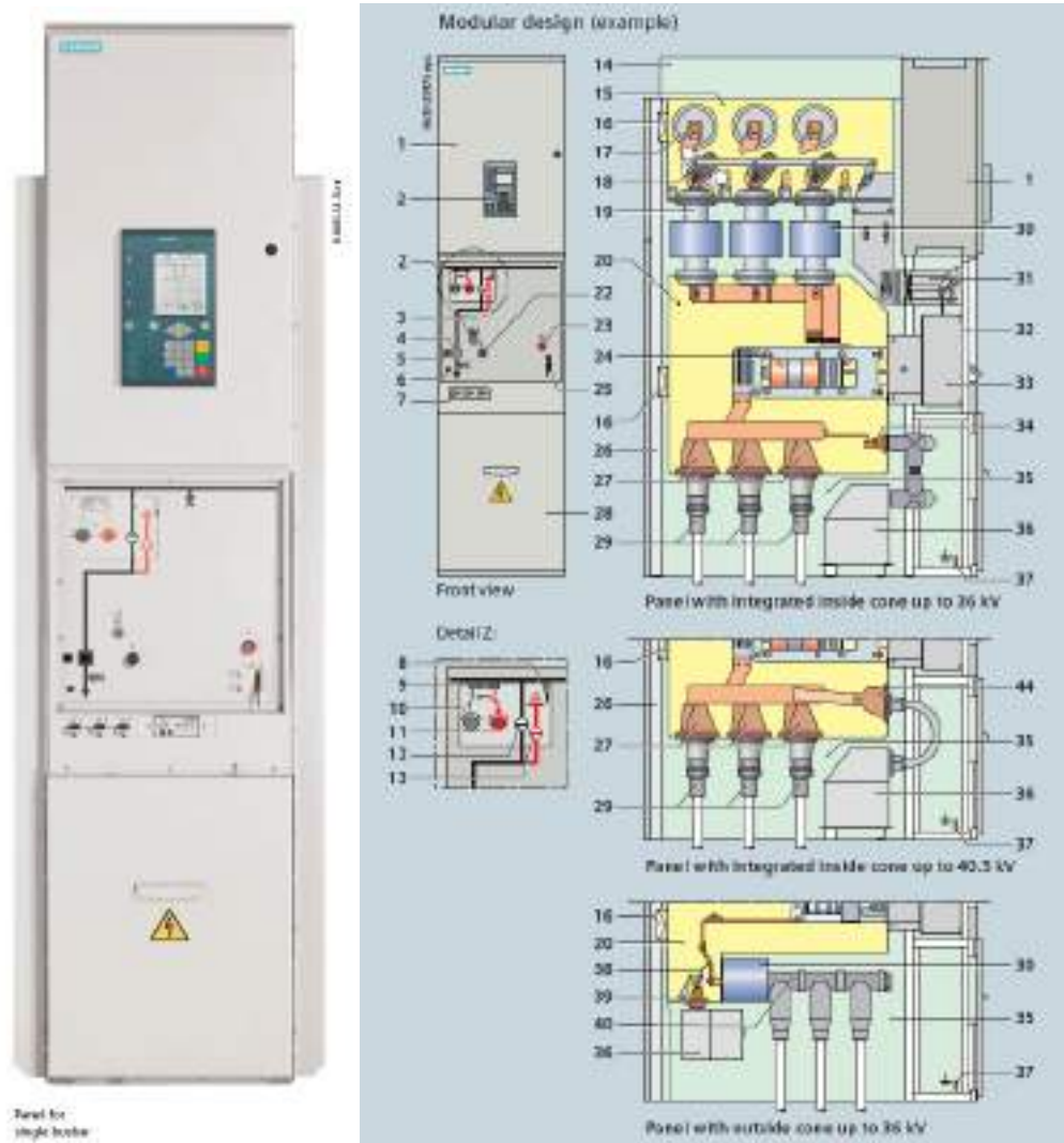
Imagen 1: Frontal e interior de celda. Permite hasta 3 botellas por fase en su conexión.
