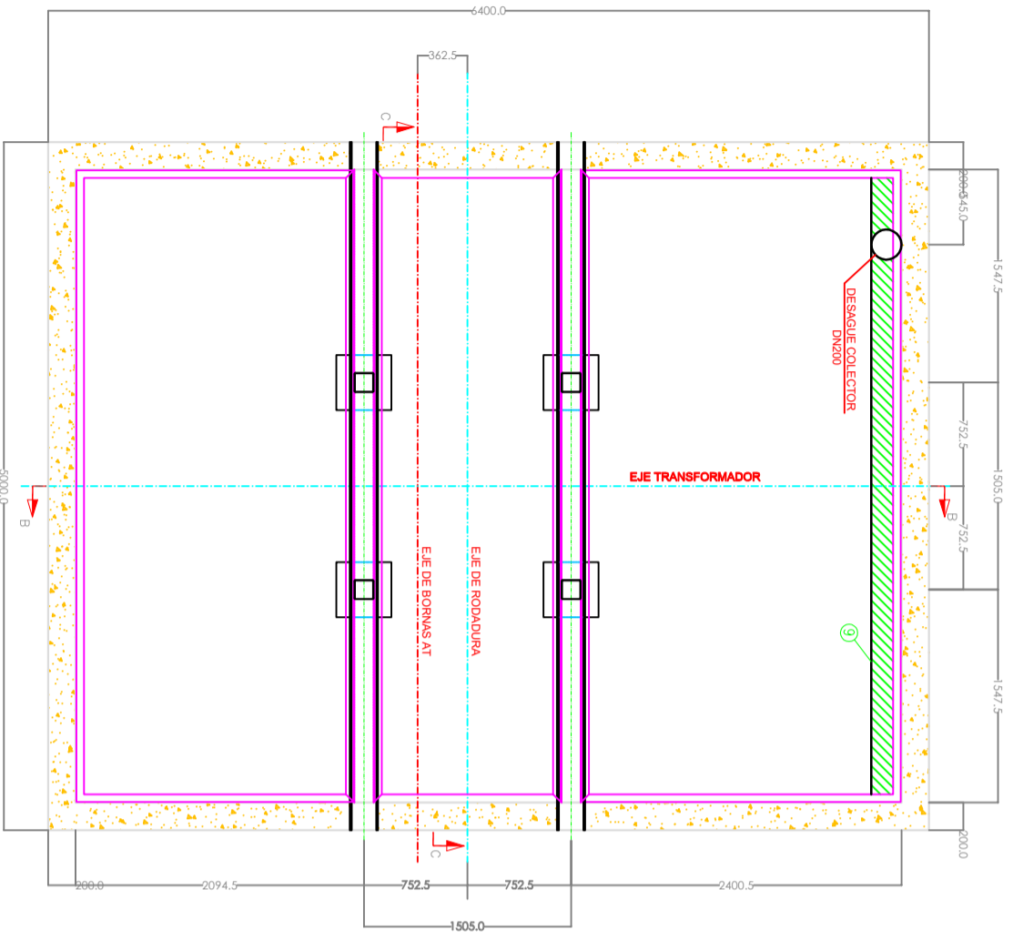
PLANTA
