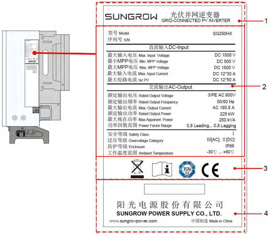
Fig.1. Nameplate
