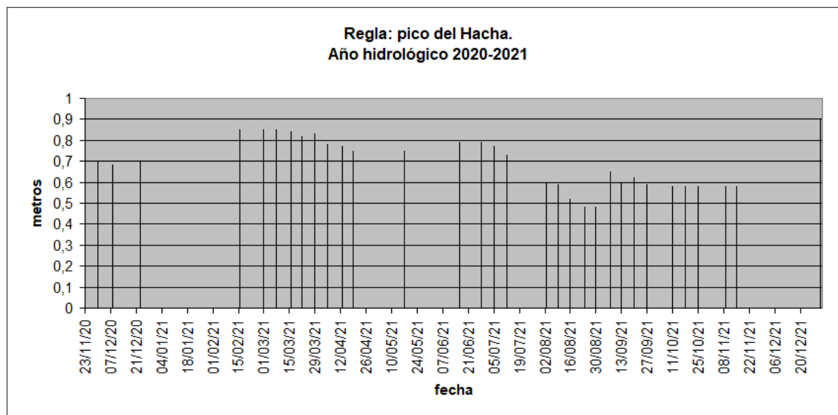
Altura de agua en la regla: pico del Hacha. Año hidrológico 2020-2021
