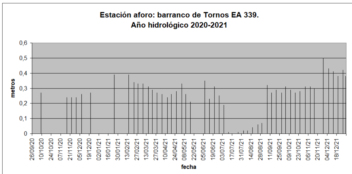
Altura de agua en la estación de aforo: barranco de Tornos. Año hidrológico 2020-2021
