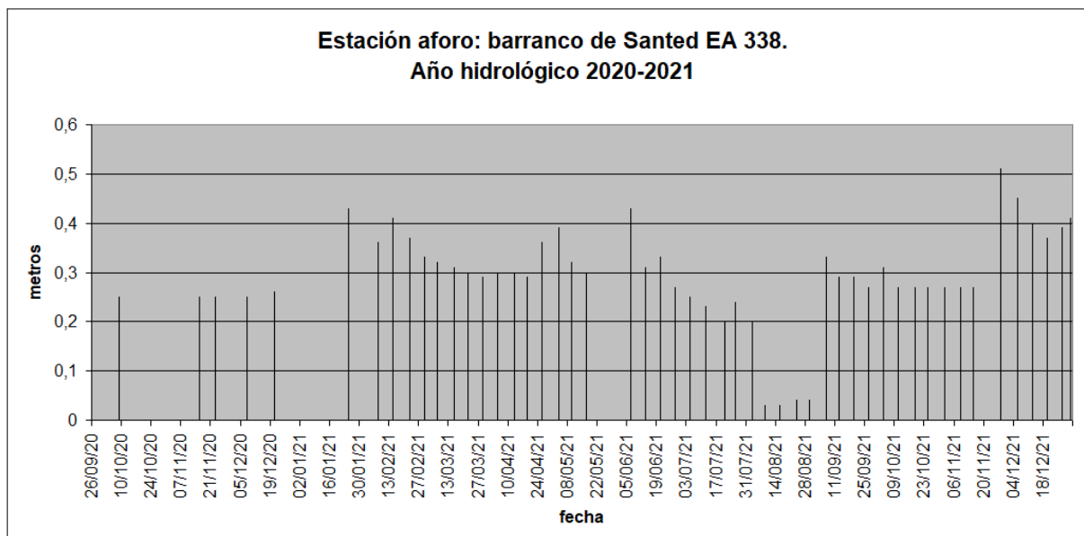
Altura de agua en la estación de aforo: barranco de Santed. Año hidrológico 2020-2021
