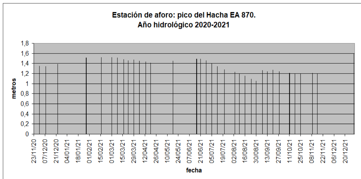
Altura de agua en la estación de aforo: pico del Hacha. Año hidrológico 2020-2021
