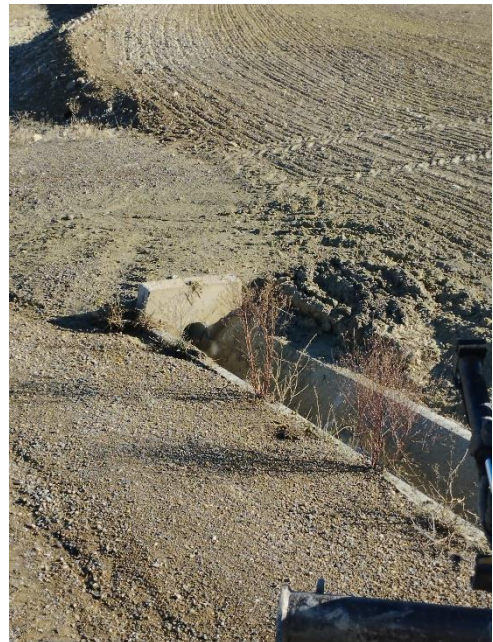
Figura 2: Vial de acceso ML4 05 antes y después de los trabajos de limpieza.
