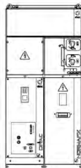
Celda Interruptor Automático (DC)
