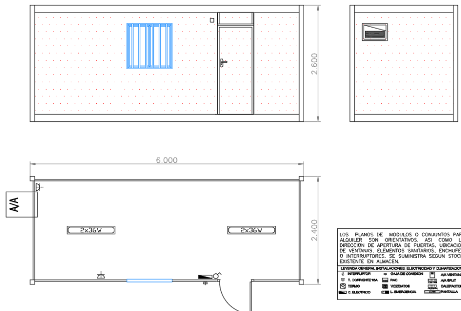
Ilustración 3: Dimensiones caseta centro de control
