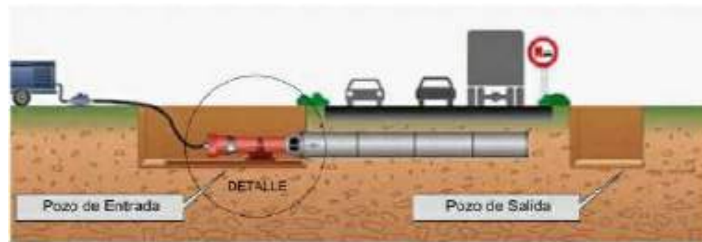
SECCION TIPO CRUCE DE VIAL CON HINCA
