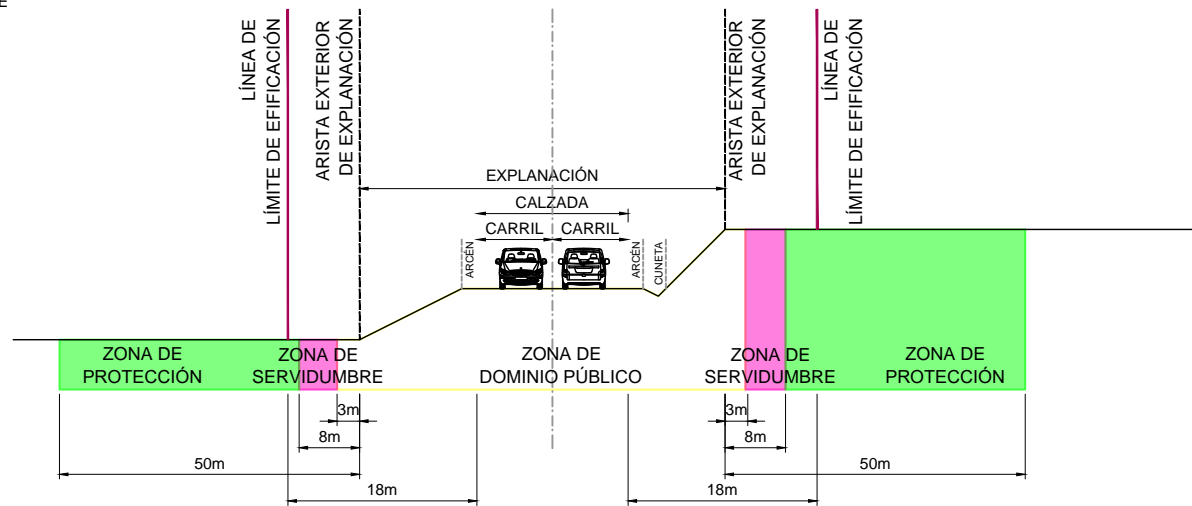
SECCION TIPO E=S/E
