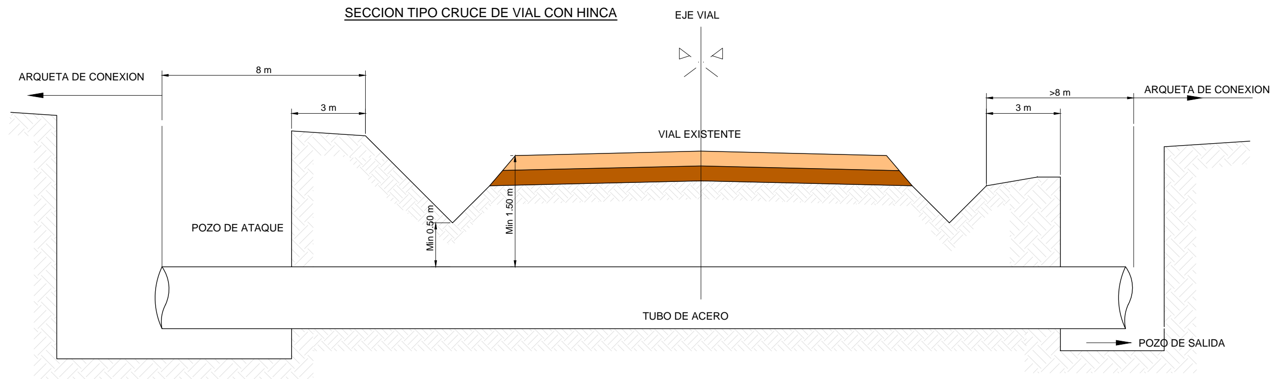
SECCIÓN TRANSVERSAL
