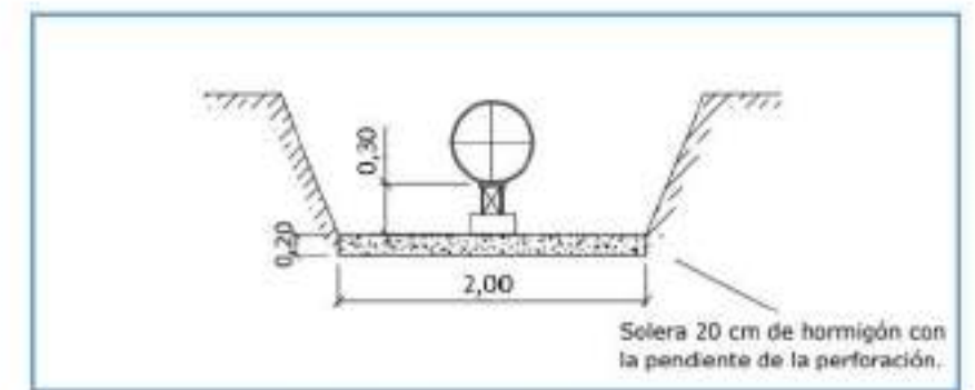
SECCIÓN TRANSVERSAL
