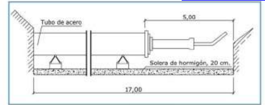
SECCIÓN LONGITUDINAL
