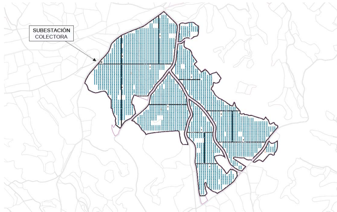
Ilustración 2. Layout Filera V (Fuente: Propia)
