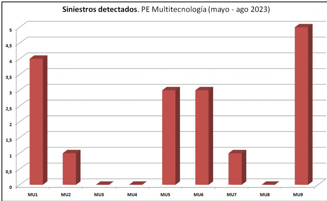
Figura 10: Gráfica de la distribución de siniestros en cada uno de los aerogeneradores del PE Multitecnología durante el presente cuatrimestre.
