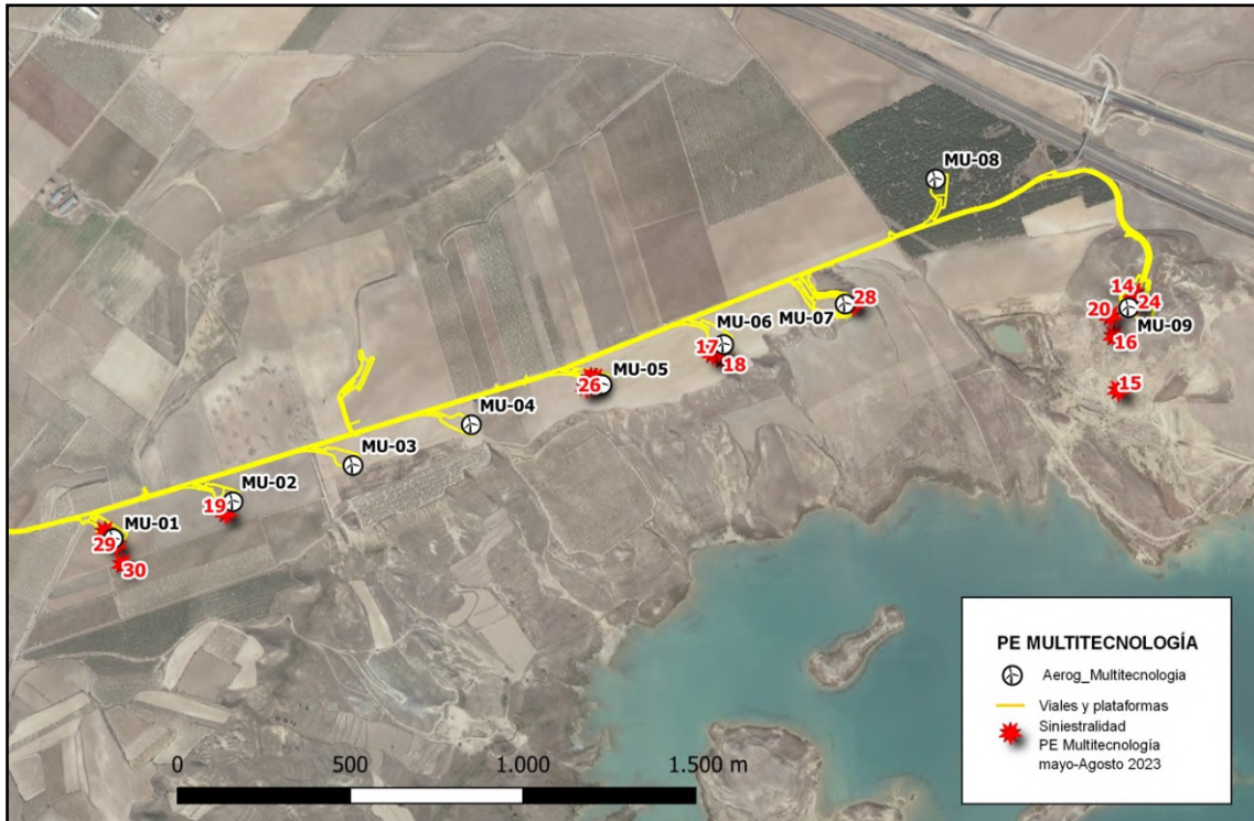
Figura 9: Plano general del PE “Multitecnología” con la localización general de los siniestros localizados en el presente cuatrimestre.
