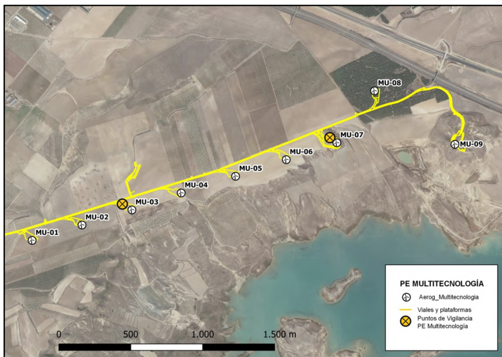
Figura 8: Plano de la localización de puntos de vigilancia para pausado preventivo en PE “Multitecnología”.
